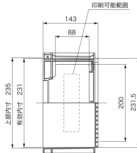
【断面視 A-A】
