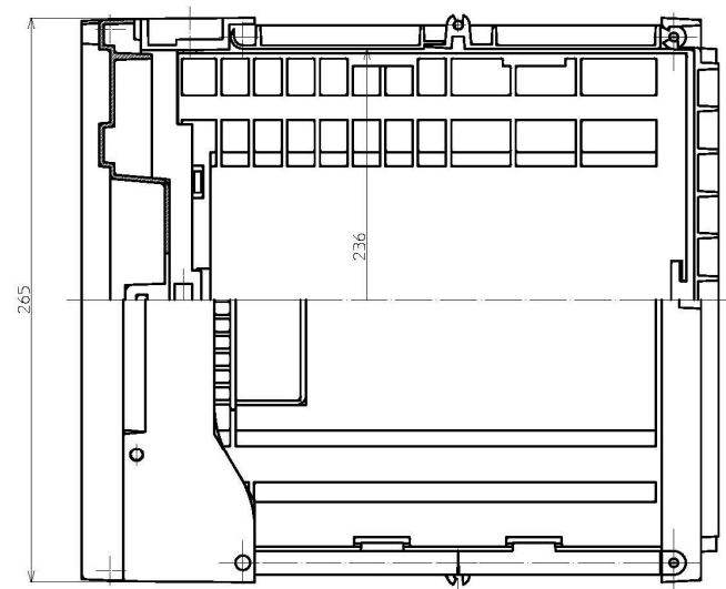
側面図
