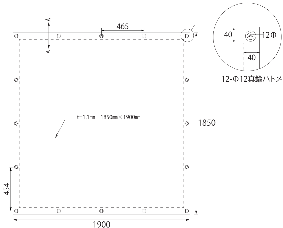
平面図
