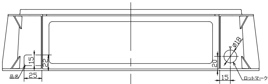
下面視
