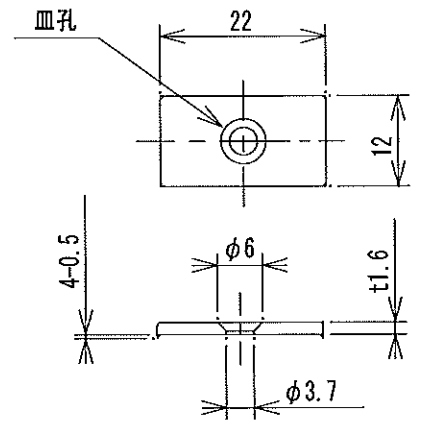
受板 M-403K
