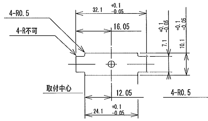
取付孔
