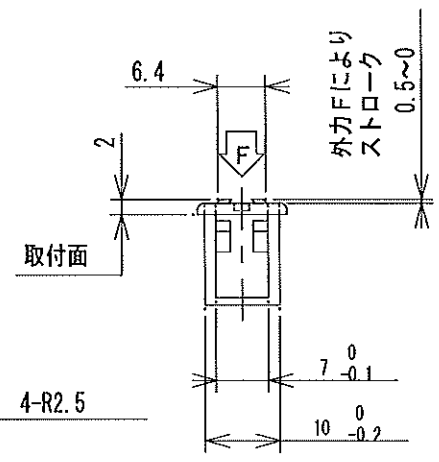
取付孔
