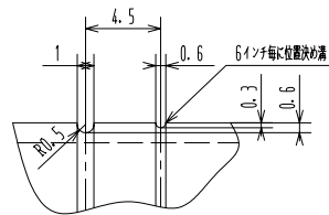
"Z" 詳細
