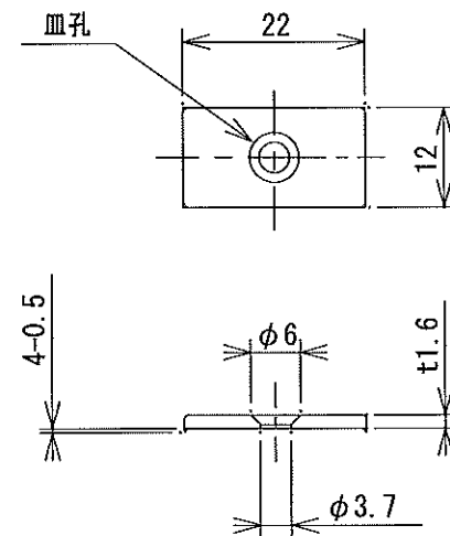
受板 M-403K
