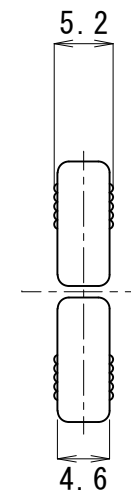
底 面 図
