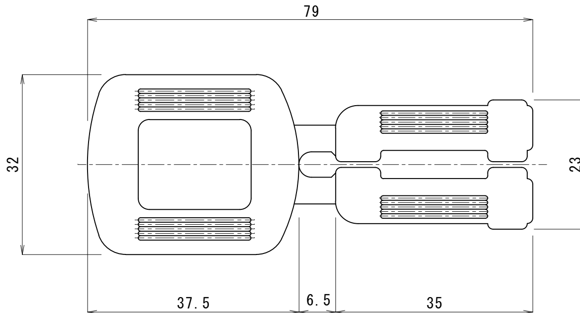
平 面 図
