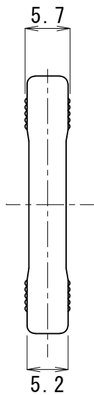
上 面 図
