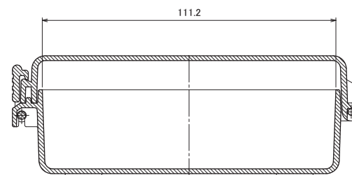
A-A' 線断面図
