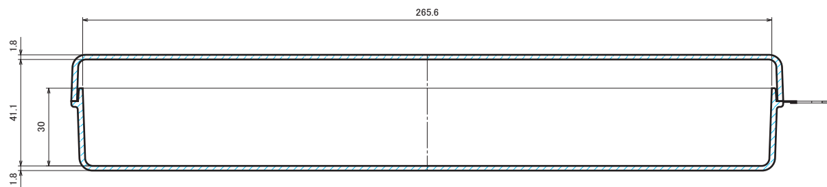
B-B' 線断面図
