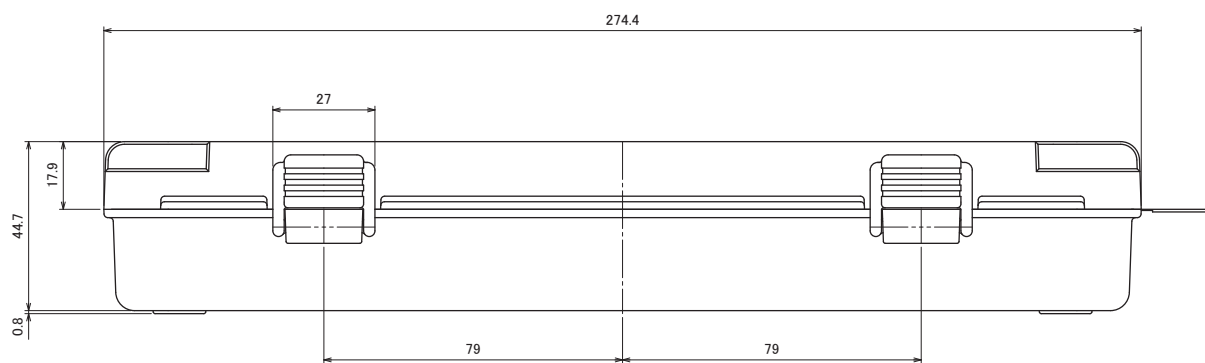
B-B' 線断面図
