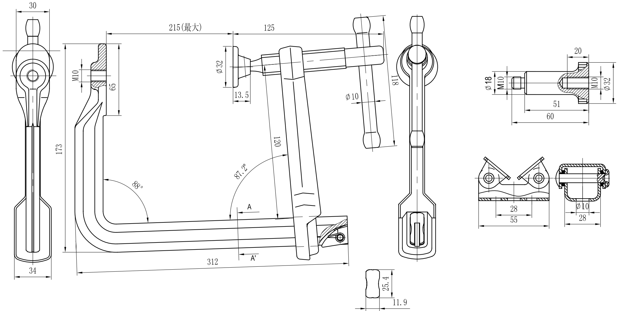
A-A'断面図
