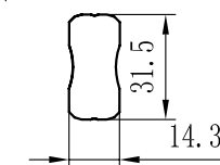
A-A'断面図
