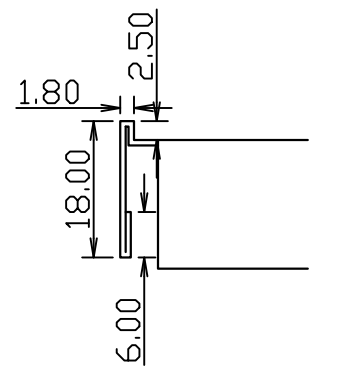
棚板開口部断面拡大図
