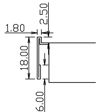
棚板開口部断面拡大図
