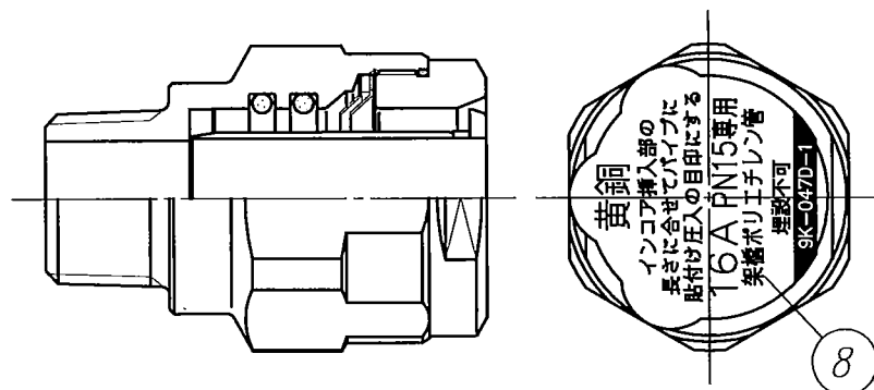
包装時組付図
