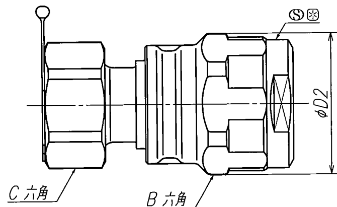
外觀図
