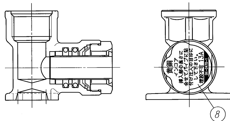
包装時組付図
