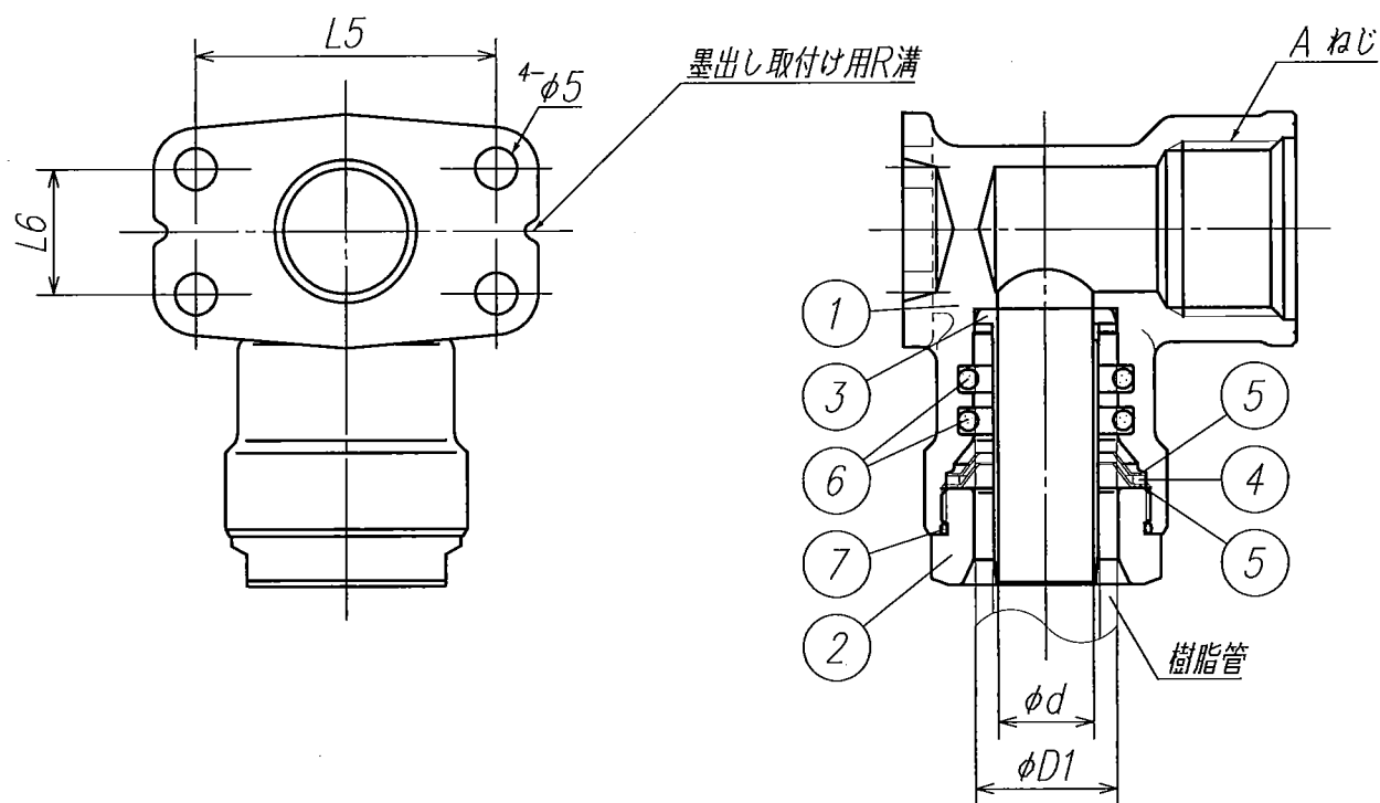
外観図
