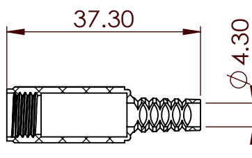
剖面圖 B-B
