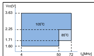
図1 : 動作温度上限とその条件
