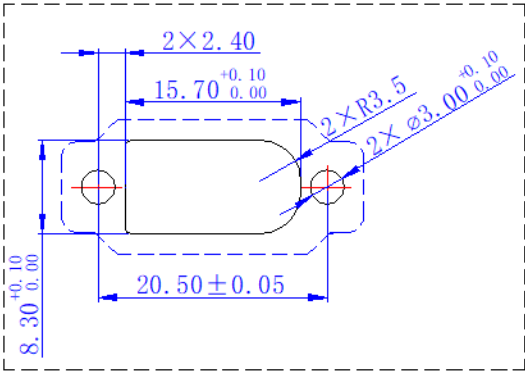
互配尺寸
