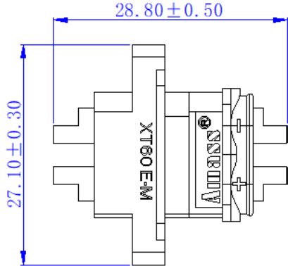
互配尺寸
