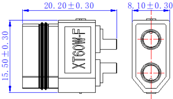
互配尺寸
