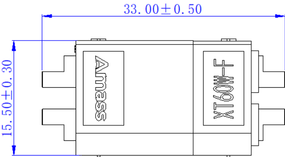
互配尺寸
