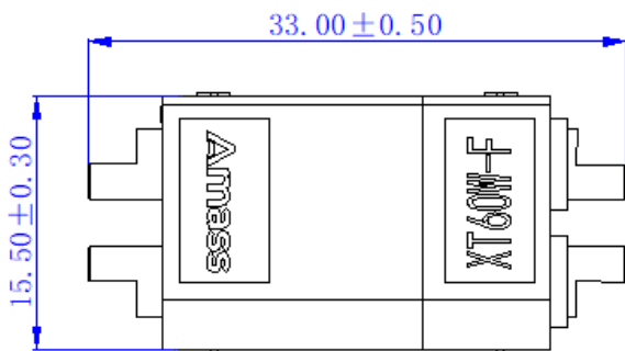
互配尺寸
