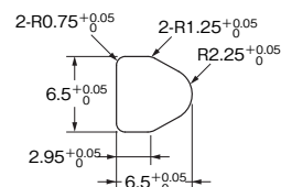
パネルカット寸法
