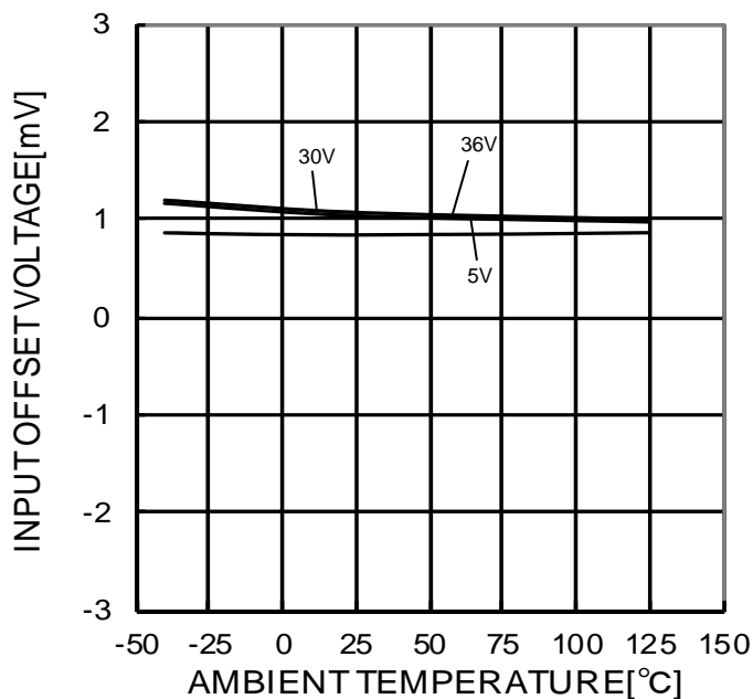
Figure 36. 入力オフセット電圧 - 温度特性
