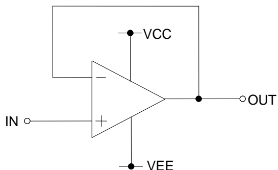
Figure 52. ボルテージフォロワ回路
