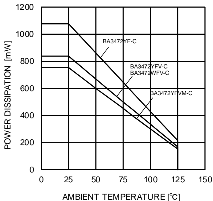
Figure 2. ディレーティングカーブ
