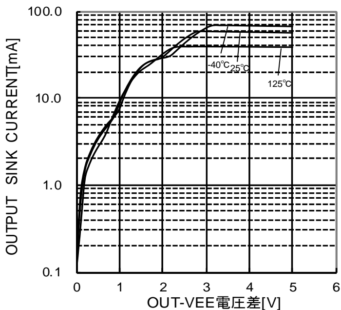
Figure 33. 出力シンク電流 - OUT-VEE 電圧差特性 (VCC/VEE=5V/0V)
