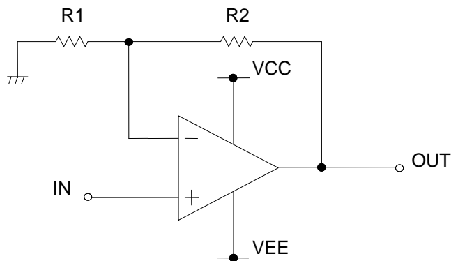
Figure 54. 非反転増幅回路
