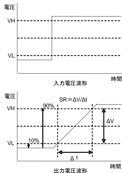
Figure 50. スルーレート測定時 入出力波形
