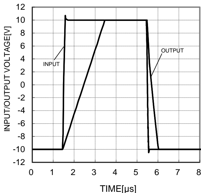
Figure 23. 大信号応答特性 (VCC/VEE=+15V/-15V, Av=0dB RL=2kΩ, CL=100pF, Ta=25°C)
