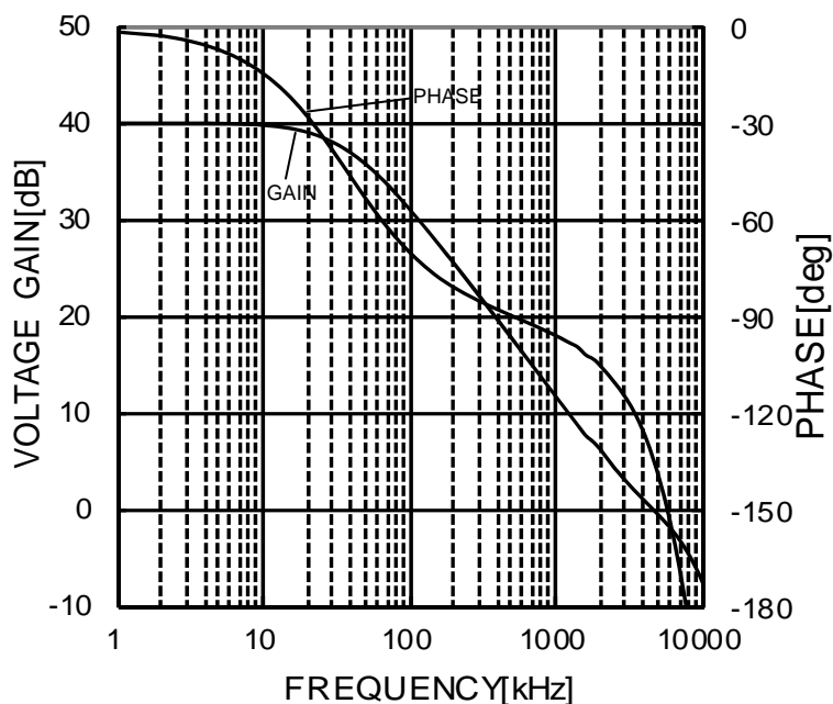
Figure 22. 電圧利得・位相 - 周波数特性 (VCC/VEE=+15V/-15V, Av=40dB RL=2kΩ, CL=100pF, Ta=25°C)
