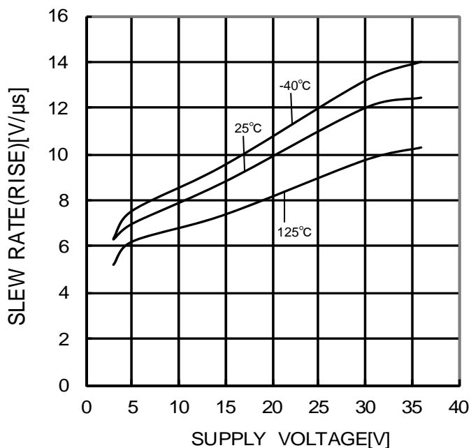
Figure 43. スルーレート(L-H) - 電源電圧特性 (RL=10kΩ)
