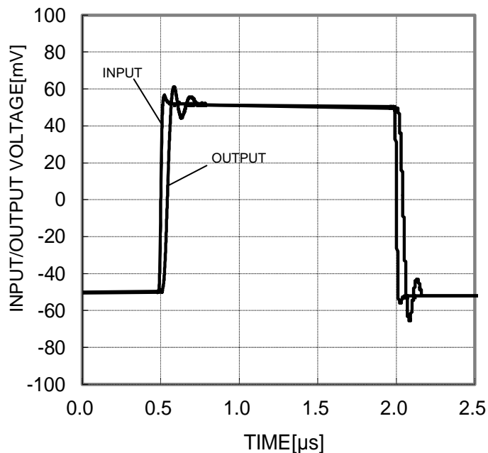
Figure 47. 小信号入出力波形 (VCC/VEE=+15V/-15V, Av=0dB RL=2kΩ, CL=100pF, Ta=25°C)
