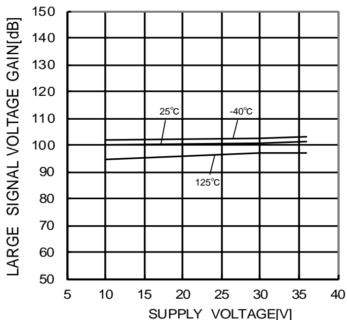
Figure 39. 大振幅電圧利得 - 電源電圧特性
