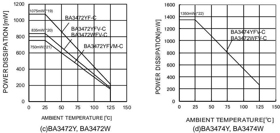
Figure 55. 熱抵抗とディレーティングカーブ
