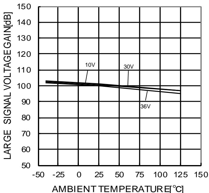
Figure 40. 大振幅電圧利得 - 温度特性
