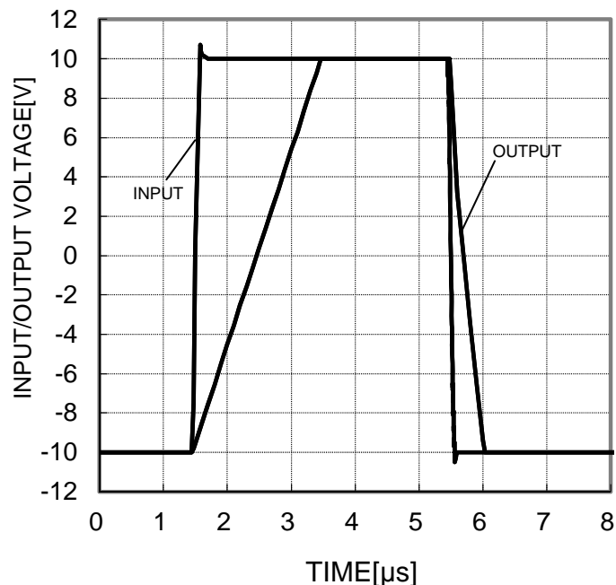
Figure 46. 大信号応答特性 (VCC/VEE=+15V/-15V, Av=0dB RL=2kΩ, CL=100pF, Ta=25°C)
