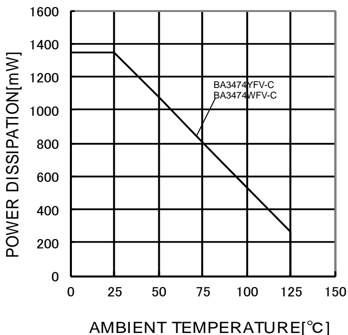
Figure 25. ディレーティングカーブ
