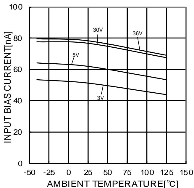
Figure 38. 入力バイアス電流 - 温度特性
