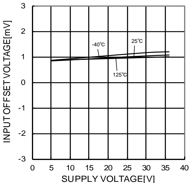
Figure 35. 入力オフセット電圧 - 電源電圧特性
