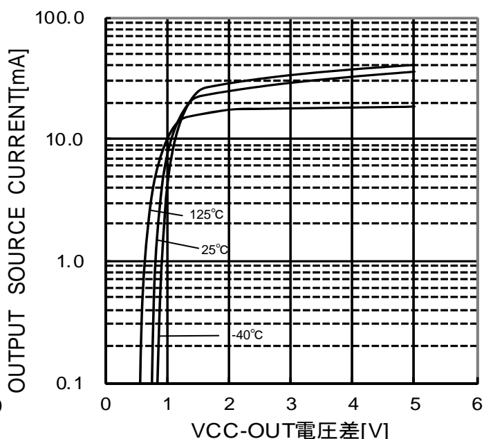
Figure 32. 出力ソース電流 - VCC-OUT 電圧差特性 (VCC/VEE=5V/0V)
