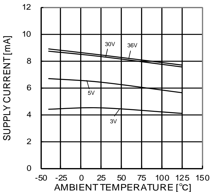
Figure 27. 回路電流 - 温度特性
