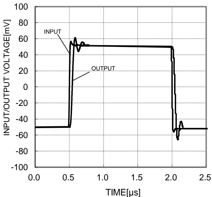
Figure 24. 小信号入出力波形 (VCC/VEE=+15V/-15V, Av=0dB RL=2kΩ, CL=100pF, Ta=25°C)
