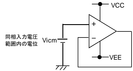
Figure 57. 未使用回路処理例
