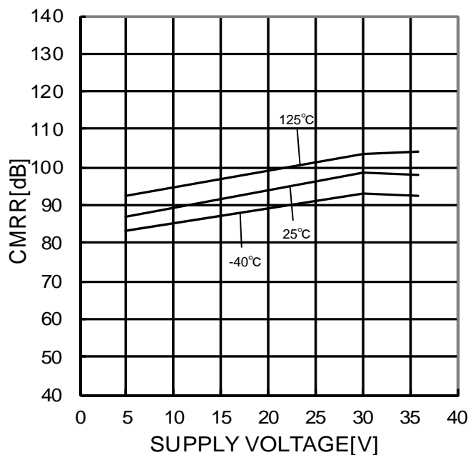
Figure 41. 同相信号除去比 - 電源電圧特性
