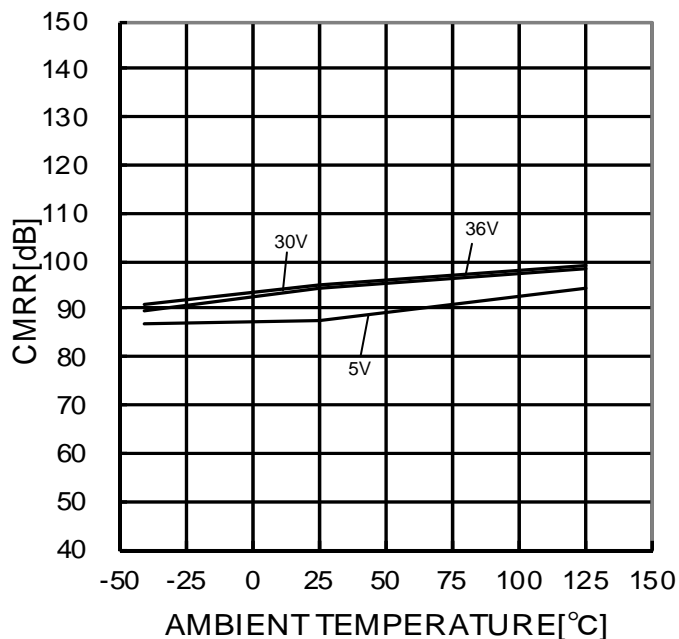
Figure 19. 同相信号除去比 - 温度特性
