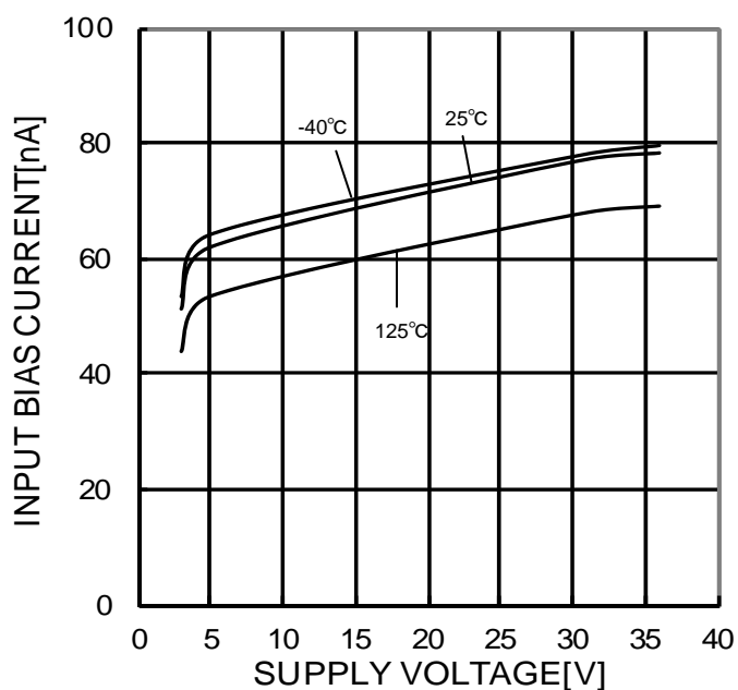
Figure 37. 入力バイアス電流 - 電源電圧特性
