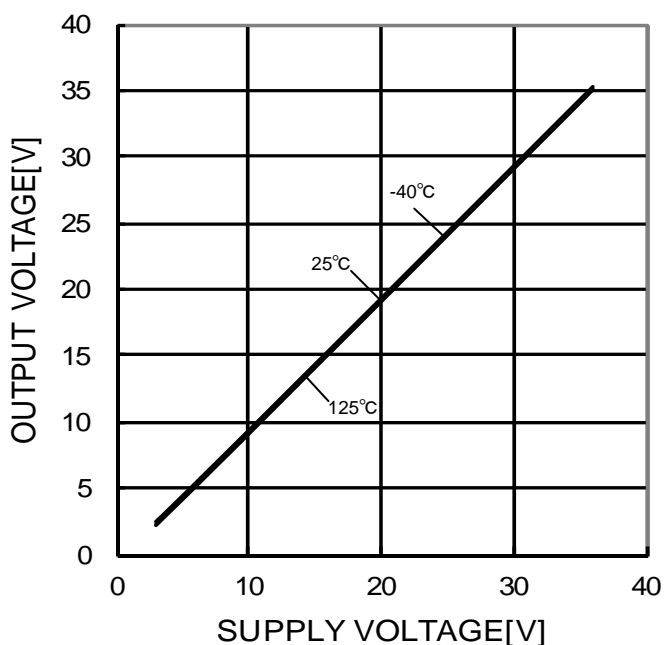
Figure 28. 最大出力電圧(High) - 電源電圧特性 (RL=10kΩ)
