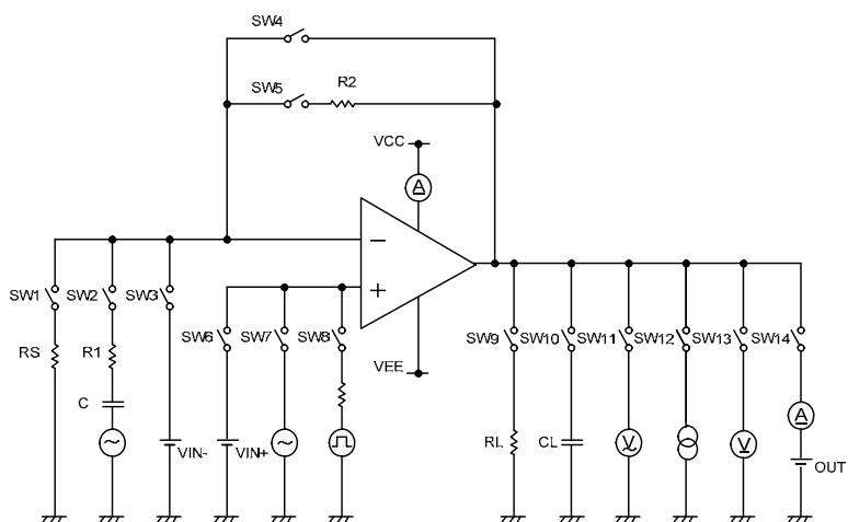
Figure 49. 測定回路 2 (1 チャンネルのみ)
