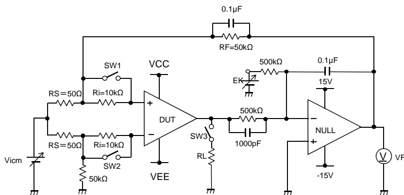
Figure 48. 測定回路 1 (1チャンネルのみ)
