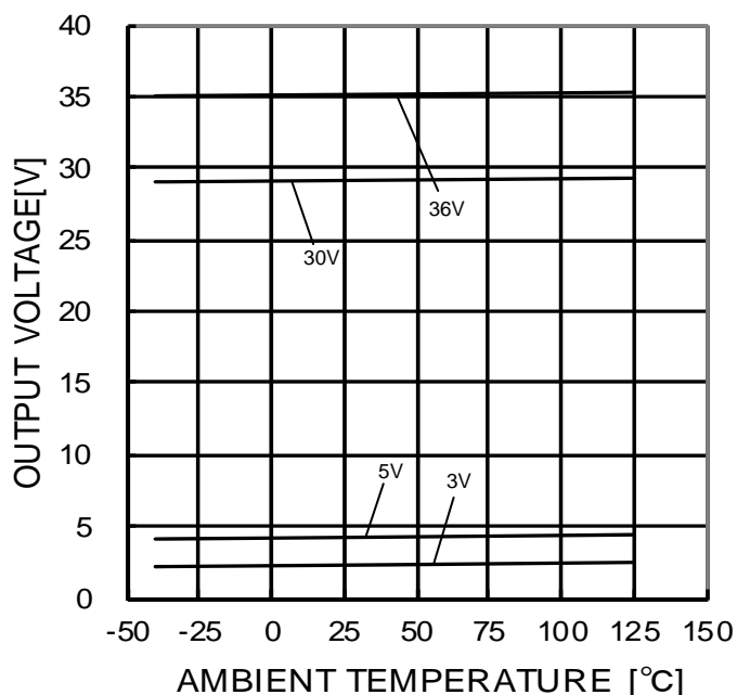
Figure 29. 最大出力電圧(High) - 温度特性 (RL=10kΩ)
