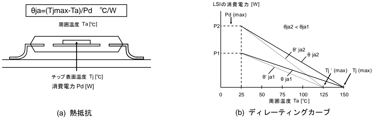
Figure 55. 熱抵抗とディレーティングカーブ
