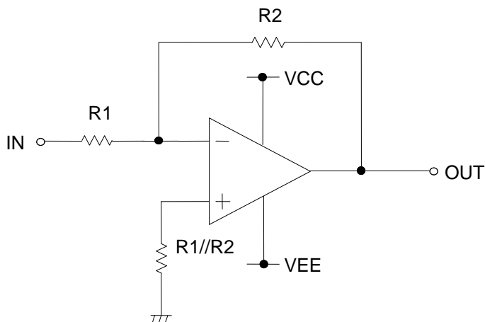
Figure 53. 反転増幅回路
