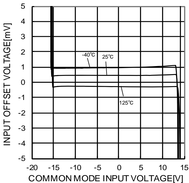
Figure 34. 入力オフセット電圧 - 同相入力電圧特性 (VCC/VEE=15V/-15V)
