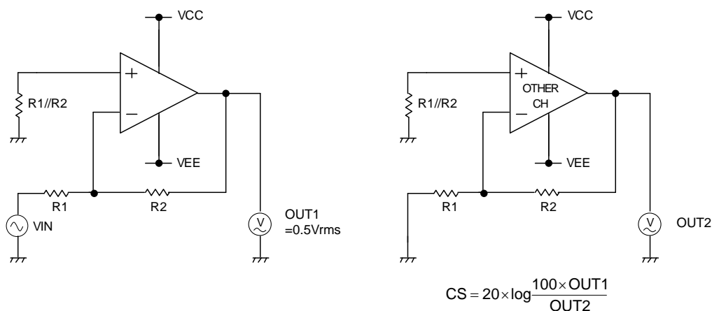
Figure 51. 測定回路 3 (チャンネルセパレーション)
