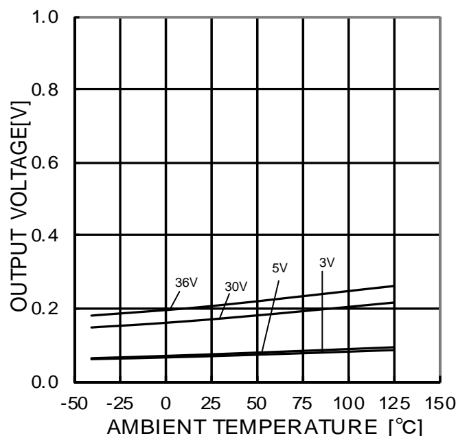
Figure 31. 最大出力電圧(Low) - 温度特性 (RL=10kΩ)
