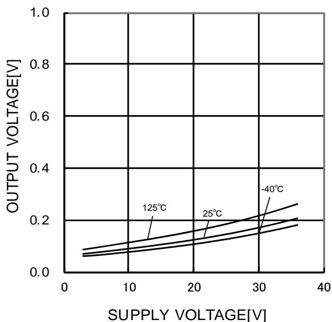
Figure 30. 最大出力電圧(Low) - 電源電圧特性 (RL=10kΩ)
