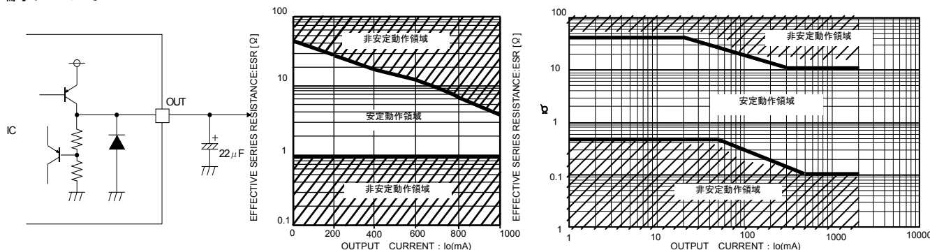
Fig.33 ESR -Io 特性(BA□□CC0,22μF)
