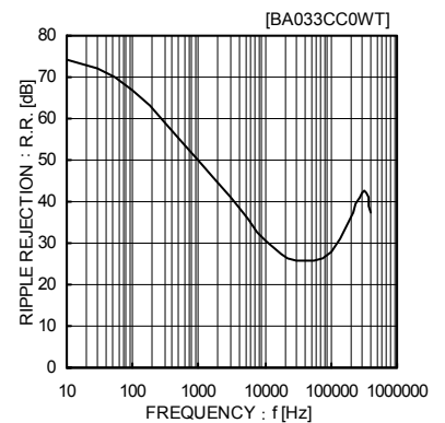
Fig.6 リプルリジェクション ( I_o=100mA )
