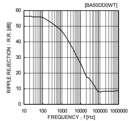
Fig.18 リプルリジェクション ( I_{out}=100mA )
