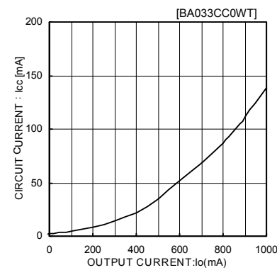
Fig.8 回路電流温度特性 ( I_{out}=0mA \rightarrow 1A )
