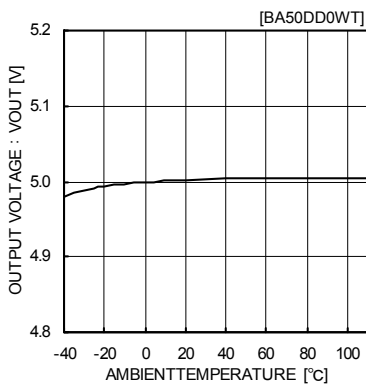
Fig.19 出力電圧温度特性
