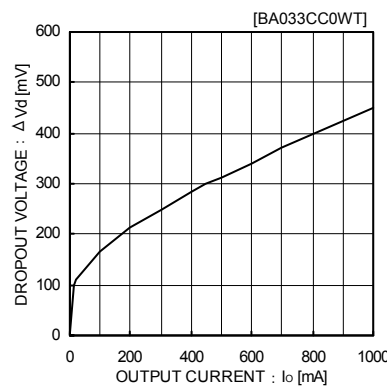
Fig.5 入出力電圧差 I_o-\Delta V_d 特性( V_{cc}=2.95V )
