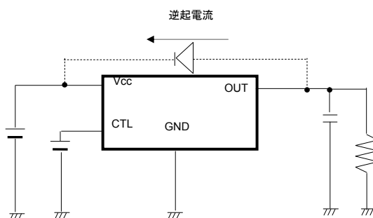
Fig.35 バイパスダイオード
