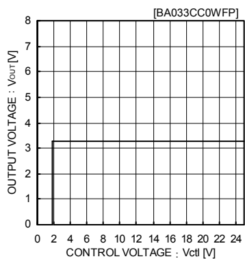
Fig.10 CTL 電圧 vs 出力電圧
