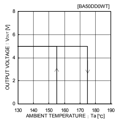
Fig.24 温度保護回路特性
