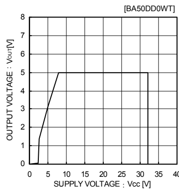
Fig.23 過電圧動作特性 ( I_o=200mA )
