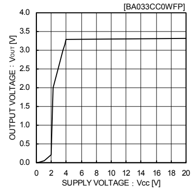
Fig.3 入力安定度 ( I_o=500mA )
