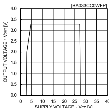
Fig.11 過電圧動作特性 ( I_o=200mA )
