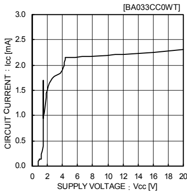
Fig.1 回路電流
