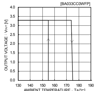
Fig.12 温度保護回路特性
