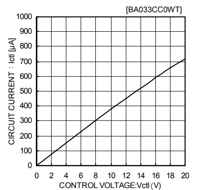
Fig.9 CTL 電圧 vs. CTL 電流
