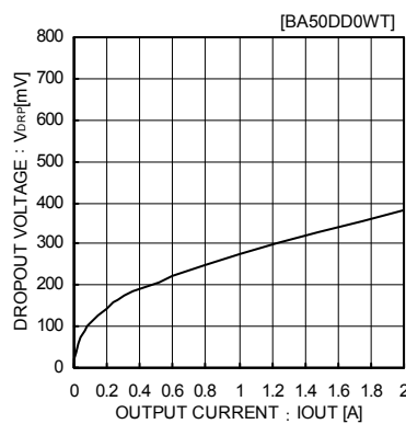
Fig.17 入出力電圧差 I_{OUT}-\Delta V_d 特性( V_{cc}=4.75V )
