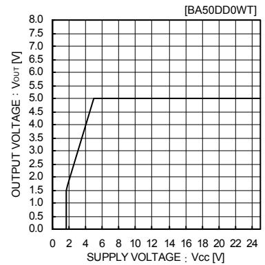
Fig.15 入力安定度 ( I_o=1A )
