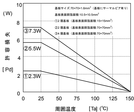
HRP-5
