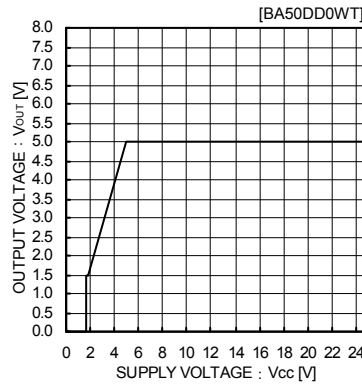
Fig.14 入力安定度 ( I_o=0mA )
