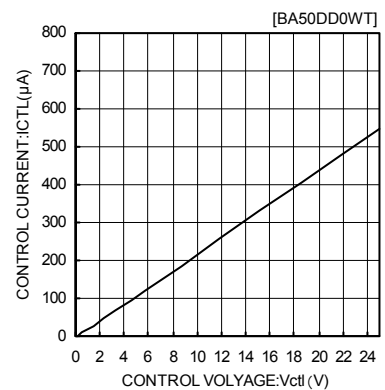
Fig.21 CTL 電圧 vs. CTL 電流
