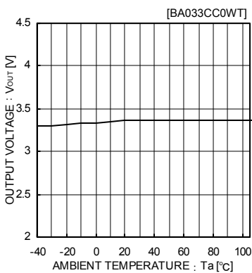
Fig.7 出力電圧温度特性
