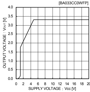
Fig.2 入力安定度
