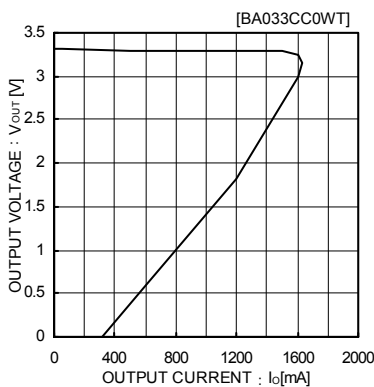
Fig.4 負荷安定度
