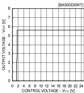
Fig.22 CTL 電圧 vs. 出力電圧
