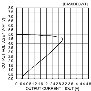
Fig.16 負荷安定度
