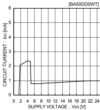
Fig.13 回路電流
