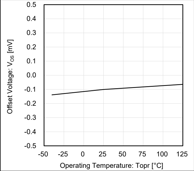
Figure 2. オフセット電圧 vs 動作温度
