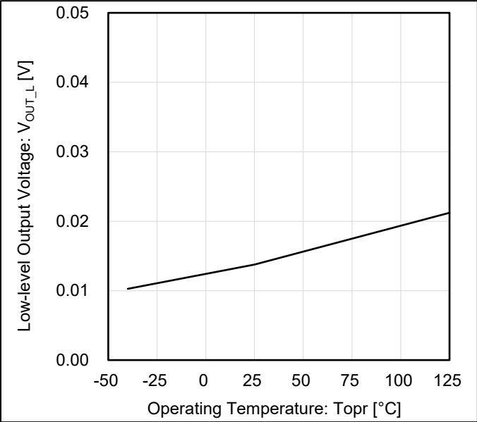
Figure 6. L 出力電圧 vs 動作温度
