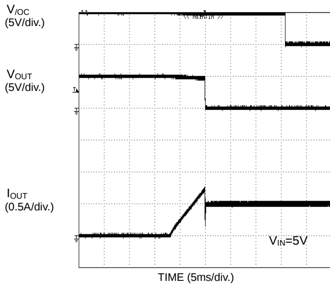
Figure 35. 過電流検出特性 ランプ出力
