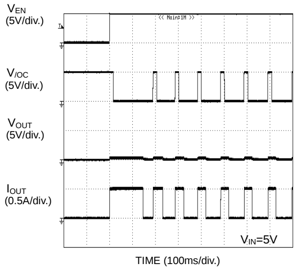
Figure 37. 過電流検出特性 ショート状態への Enable
