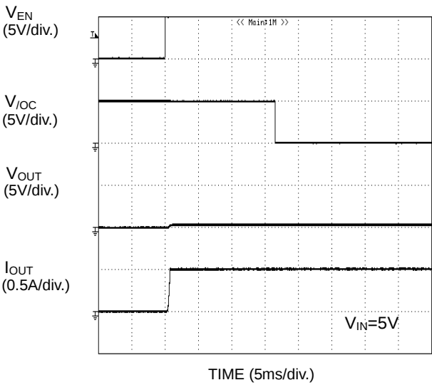
Figure 36. 過電流検出特性 ショート状態への Enable
