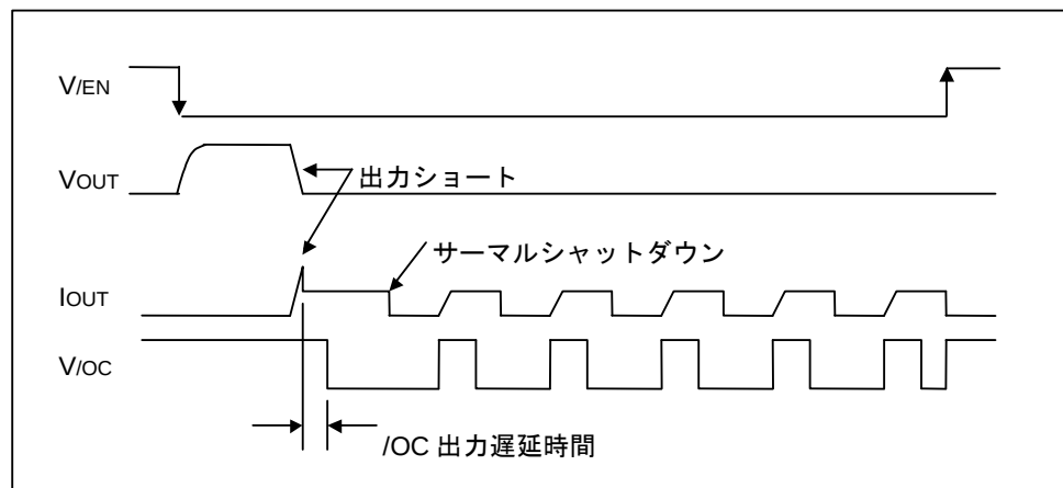
Figure 43. 過電流検出、サーマルシャットダウンタイミング (BD2247G)
