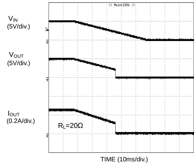
Figure 40. UVLO 特性 V_{IN} 下降時
