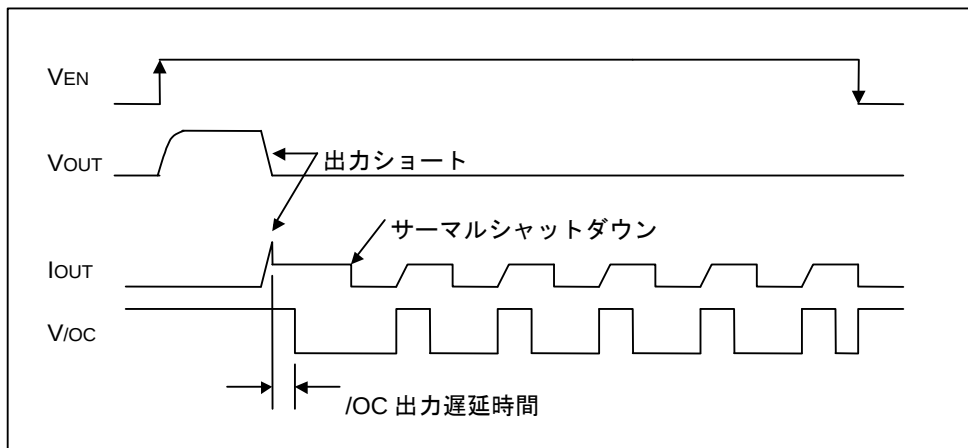
Figure 42. 過電流検出、サーマルシャットダウンタイミング (BD2246G)
