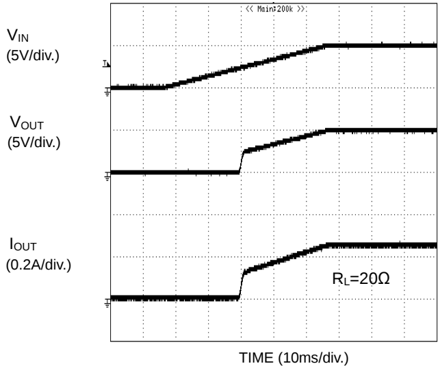
Figure 39. UVLO 特性 V_{IN} 上昇時
