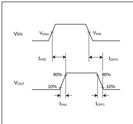
Figure 2. 出力立上り時間、出力立下り時間 (BD2246G)
