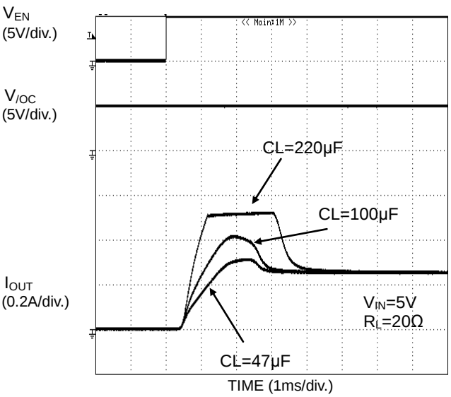
Figure 34. 突入電流特性
