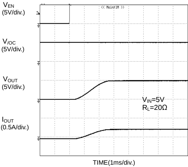
Figure 32. 出力立ち上がり特性
