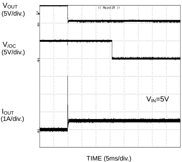
Figure 38. 過電流検出特性 Enable 時に出力 1Ω ショート
