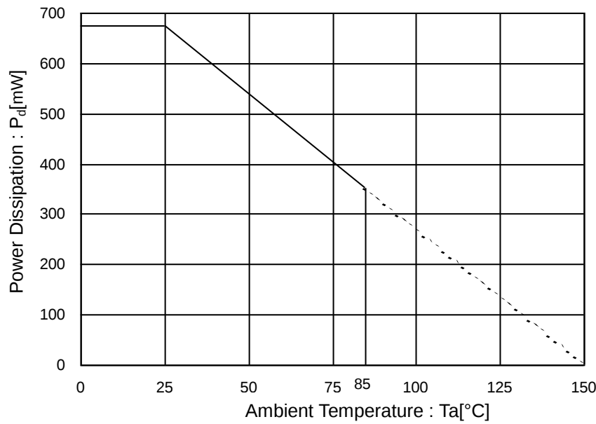
Figure 44. パッケージ熱損失について (Pd-Ta Curve)
