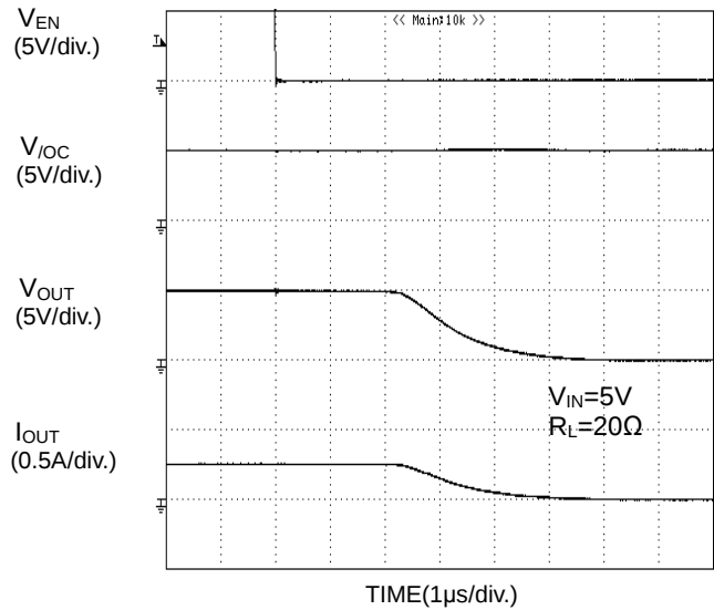
Figure 33. 出力立ち下がり特性
