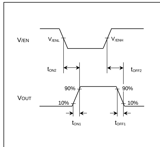
Figure 3. 出力立上り時間、出力立下り時間 (BD2247G)
