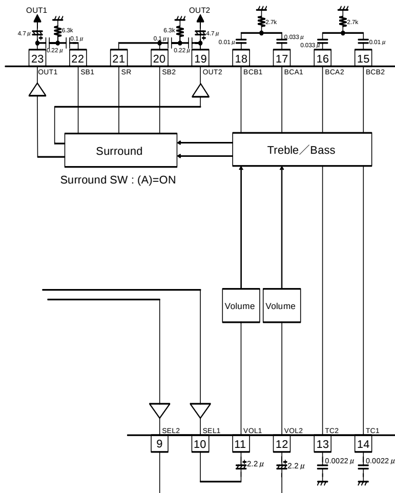
Figure 34. 簡易 3 バンド使用時の応用回路例
