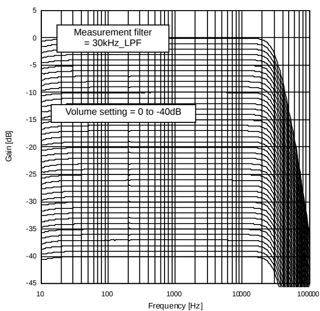
Figure 8. Volume 減衰量 1
