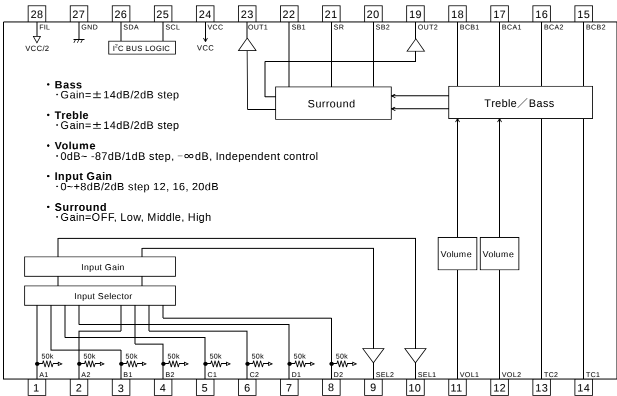
Figure 3. ブロック図
