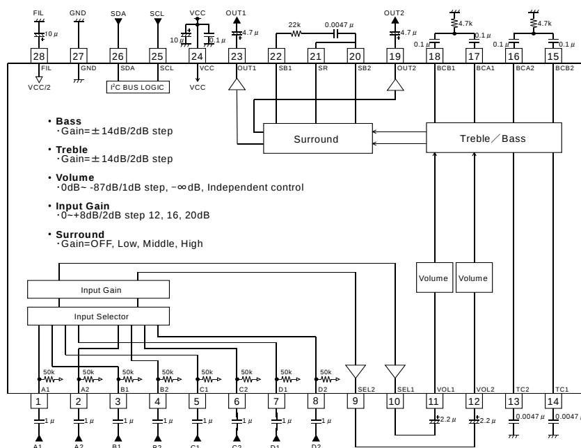
Figure 1. 応用回路例
