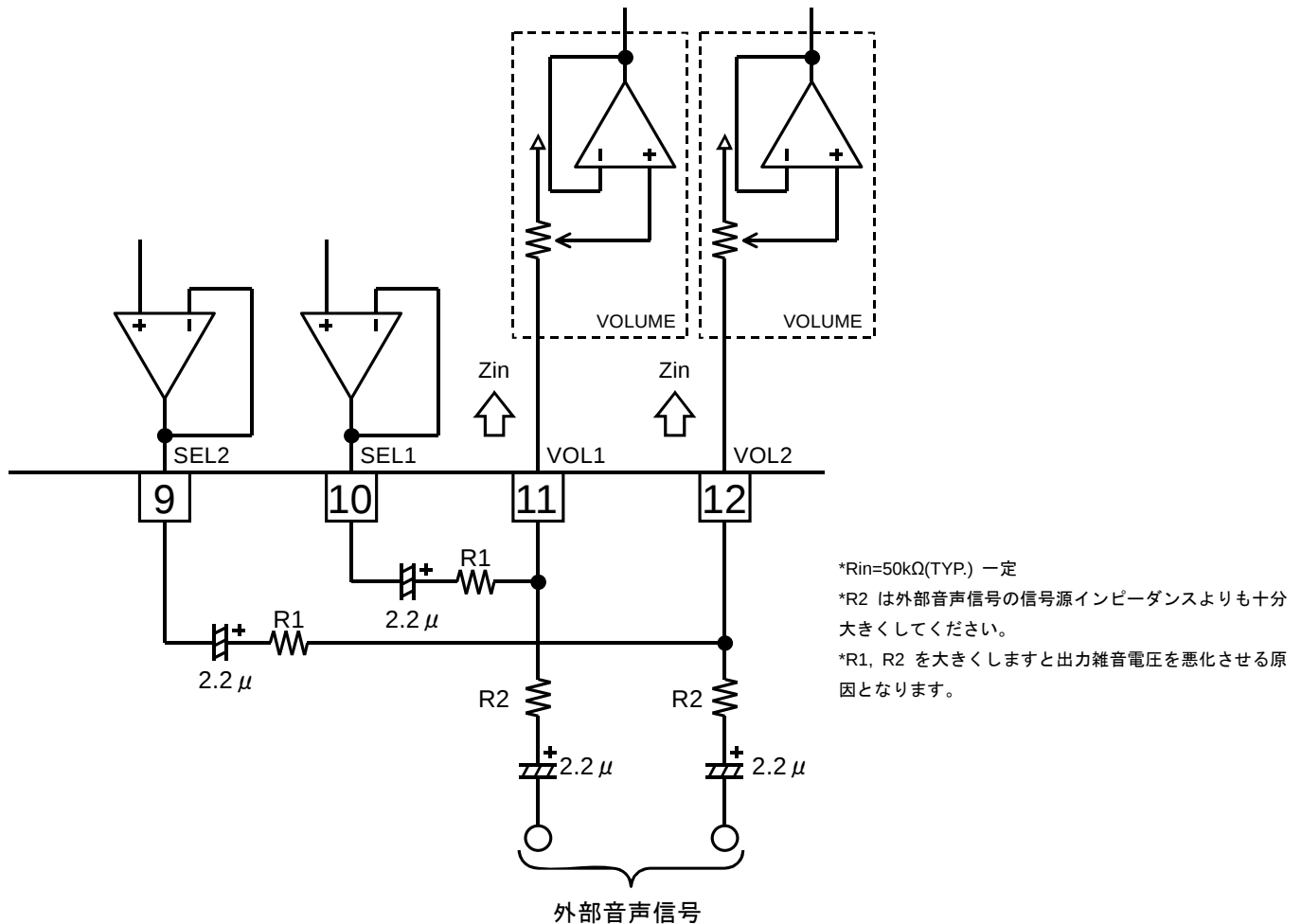
Figure 38. マイク入力使用時の応用回路例
