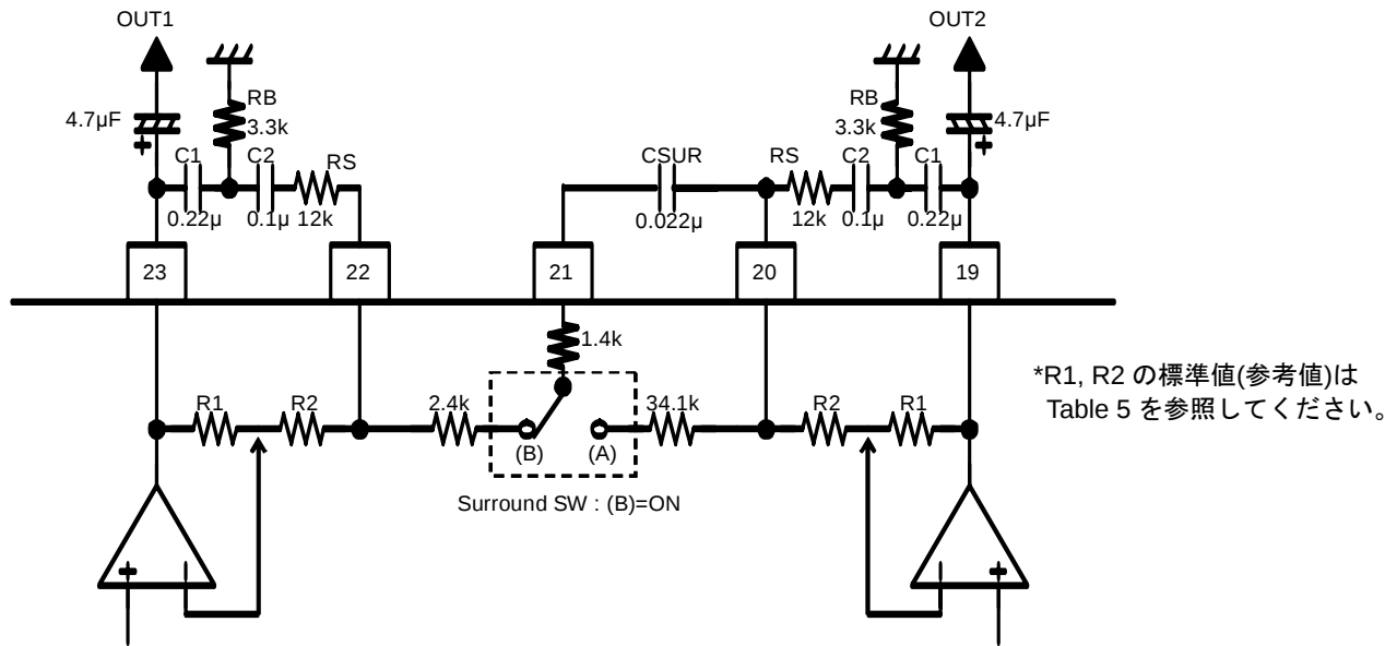
Figure 25. Bass Boost &amp; Surround 使用時の応用回路例
