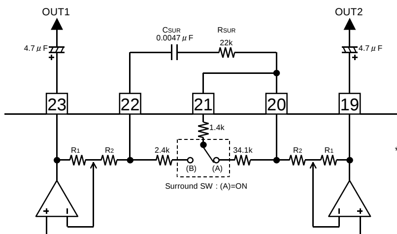
Figure 30. Surround 使用時の応用回路例
