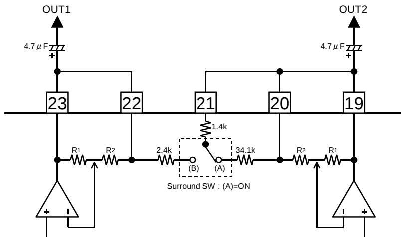
Figure 36. 付加機能未使用時の応用回路例
