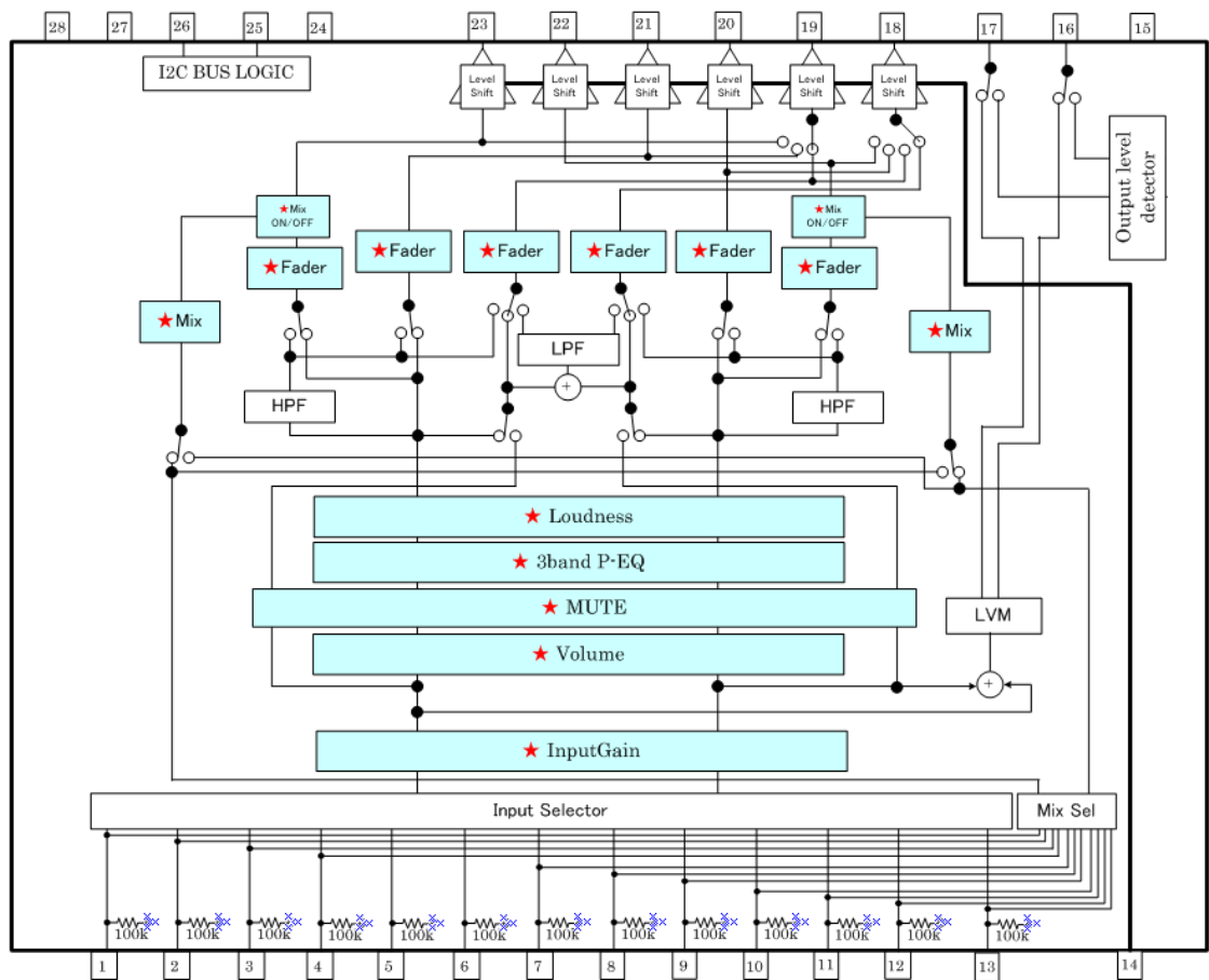
Figure 3. ブロック図
