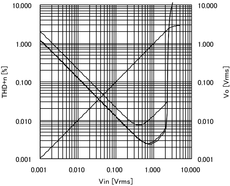
Figure 7. THD vs Vin / Vo
