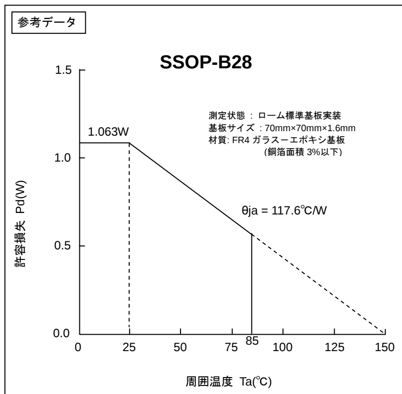
Figure 27. 熱軽減率曲線
