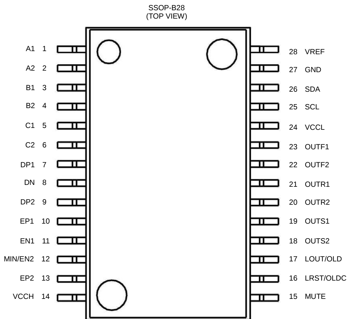
Figure 2. 端子配置図
