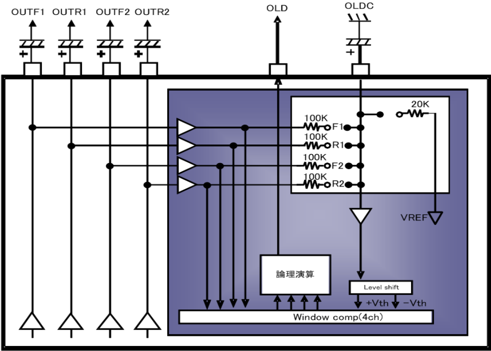
Figure 25. 出力レベル検出回路ブロック図
