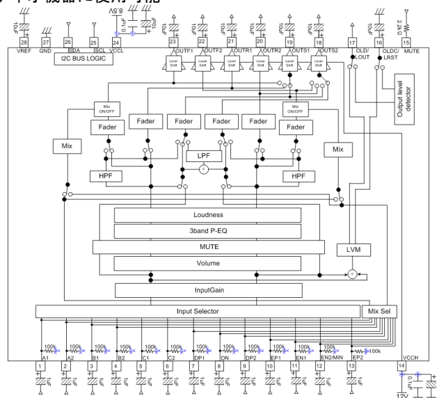
Figure 1. 応用回路例
