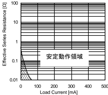
出力コンデンサ ESR VS 出力負荷(I OUT )特性 (参考データ)
