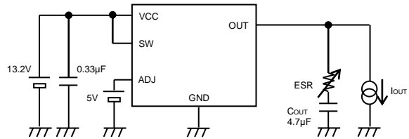
注意: 参考データ測定回路図
