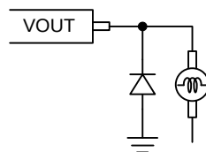
Figure 48. 応用回路例 3
