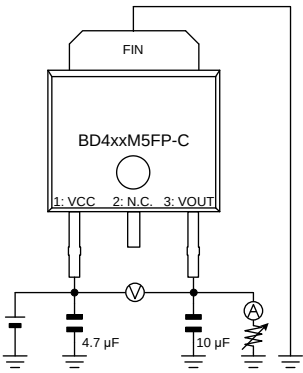
Figure 11、29 の測定回路図
