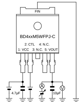
Figure 10、28 の測定回路図
