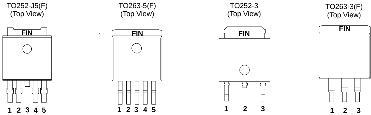
Figure 3. 端子配置図
