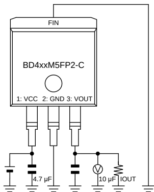
Figure 9、27 の測定回路図
