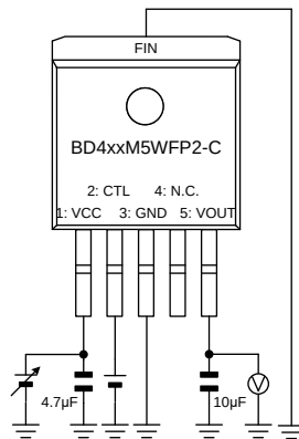
Figure 6、8、14、15、 Figure 24、26、32、33 の測定回路図
