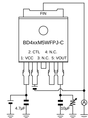
Figure 13、31 の測定回路図
