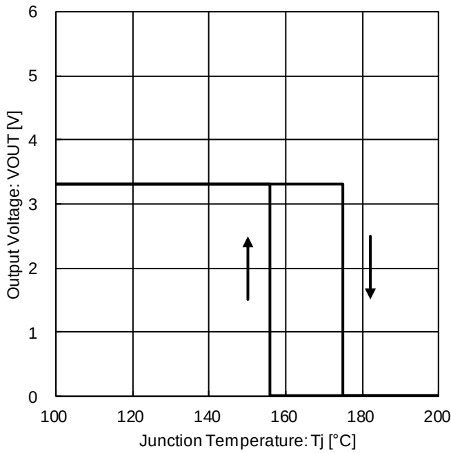
Figure 14. 温度保護回路特性
