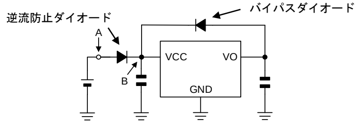
Figure 50. 推薦ダイオード使用例
