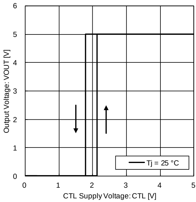
Figure 37. CTL 端子 ON / OFF モード電圧 (Tj = 25 °C)
