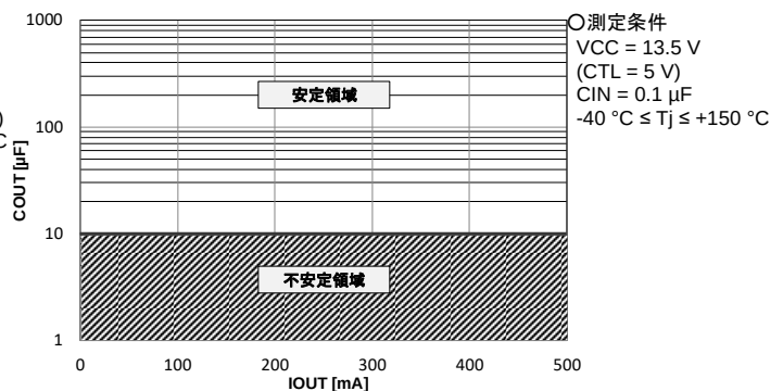
Figure 42. C OUT (Typ.) vs. 出力電流 (I OUT )
