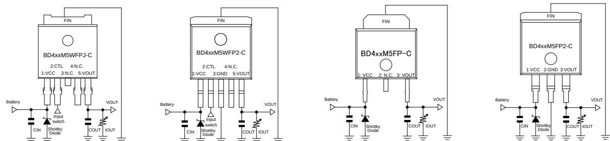
Figure 47. 応用回路例 2
