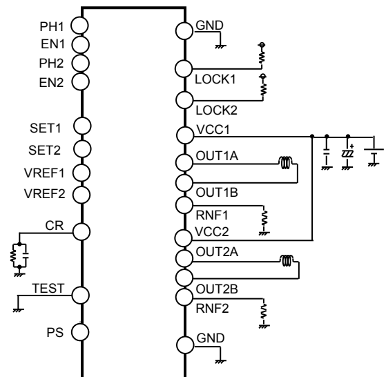
Figure 2. アプリケーション回路図
