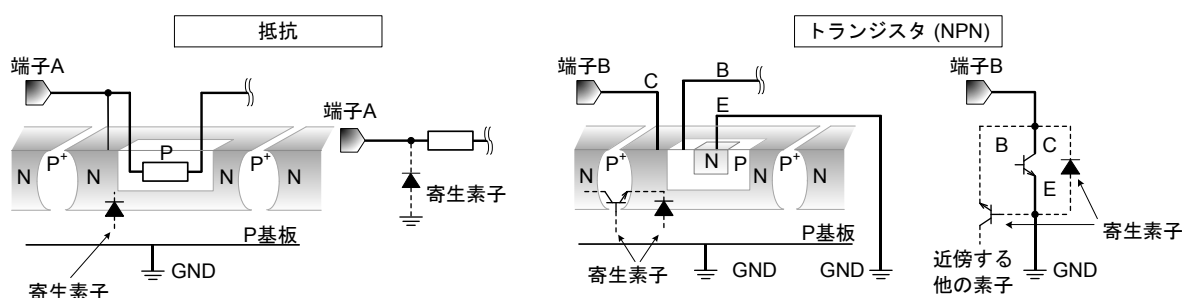
Figure 6. モノリシック IC 構造例
