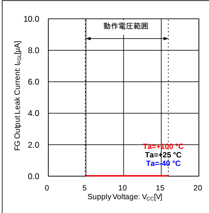
Figure 19. FG 出力リーク電流 vs 電源電圧
