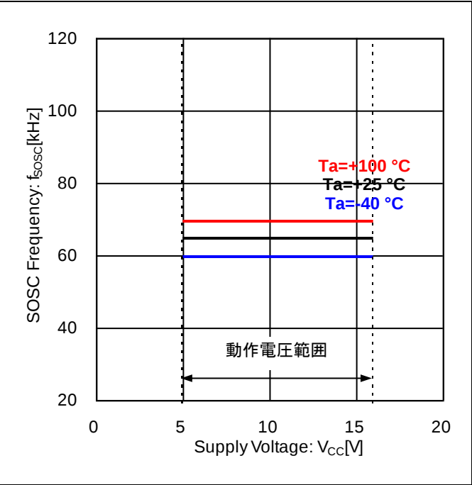
Figure 9. SOSC 発振周波数 vs 電源電圧 ( C_{sosc}=680\text{ pF} )
