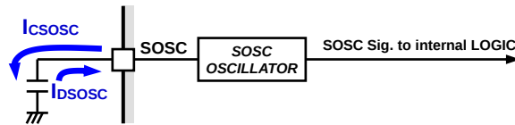
Figure 28. SOSC 端子と内部回路
