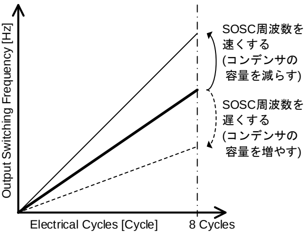
Figure 27. 出力切り替え周波数 vs 電気角周期 (強制同期起動区間)
