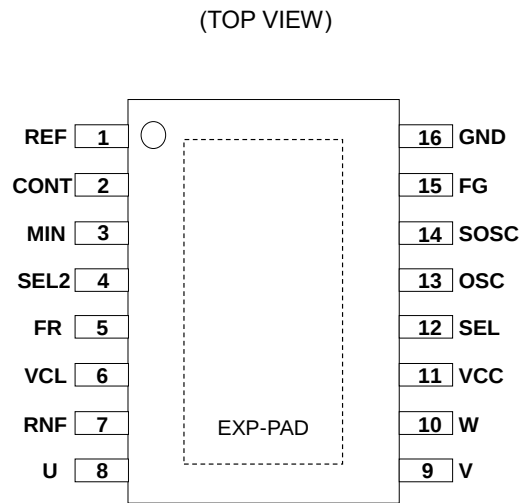
Figure 1. 端子配置図
