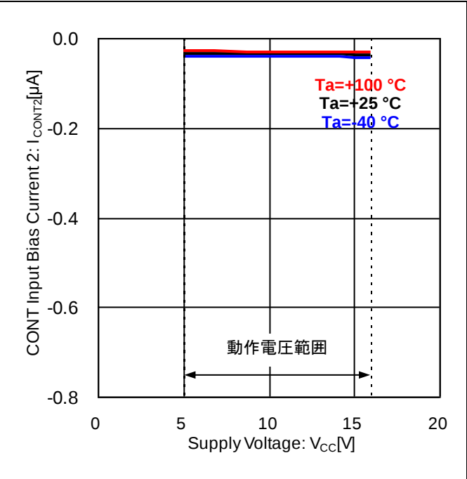
Figure 11. CONT 入力バイアス電流 2 vs 電源電圧
