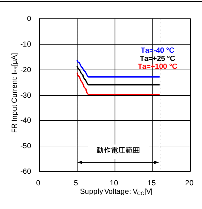
Figure 25. FR 入力電流 vs 電源電圧 ( V_{FR}=0 V)
