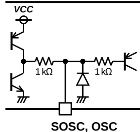
6. SOSOC, OSC 端子
