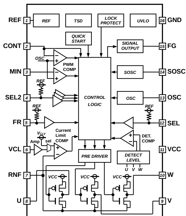
Figure 2. ブロック図
