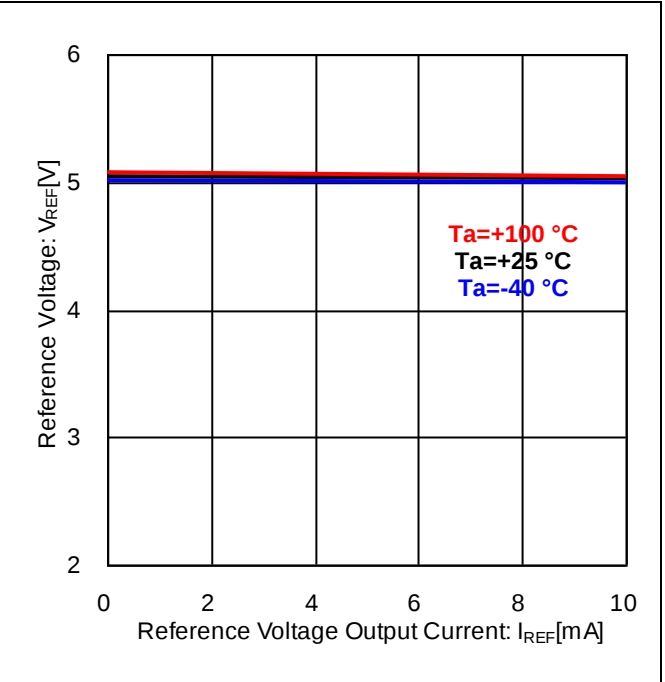
Figure 7. 基準電圧 vs 基準電圧出力電流 ( V_{CC}=12\text{ V} )
