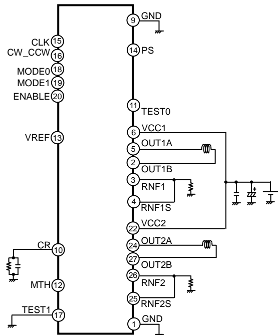
Figure.1 BD63511EFV アプリケーション回路図
