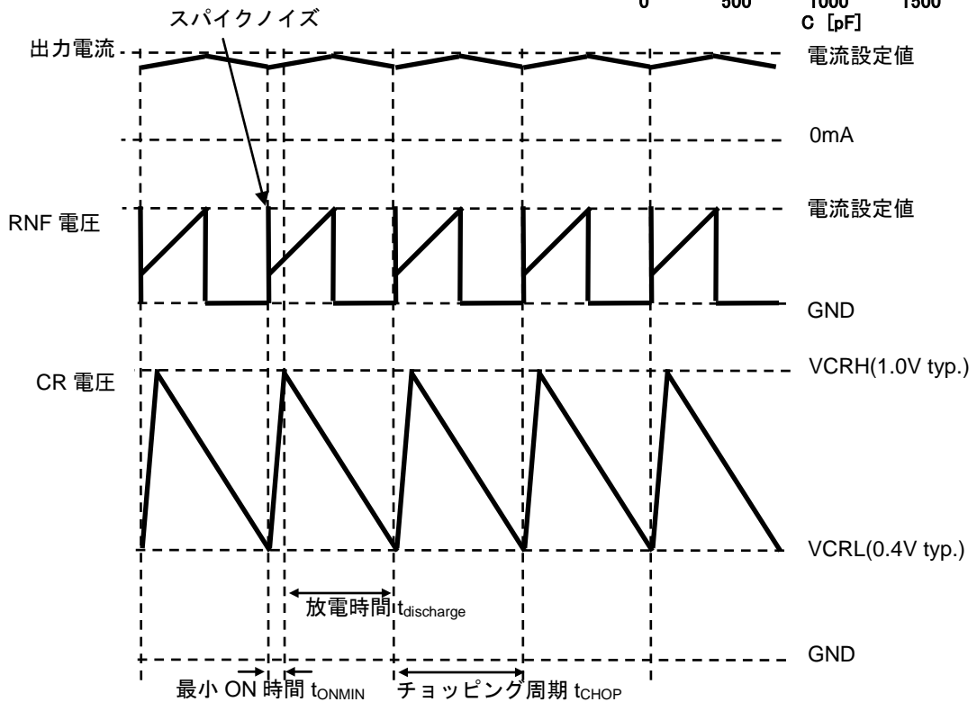
Figure.4 CR 電圧、RNF 電圧、出力電流タイミングチャート
