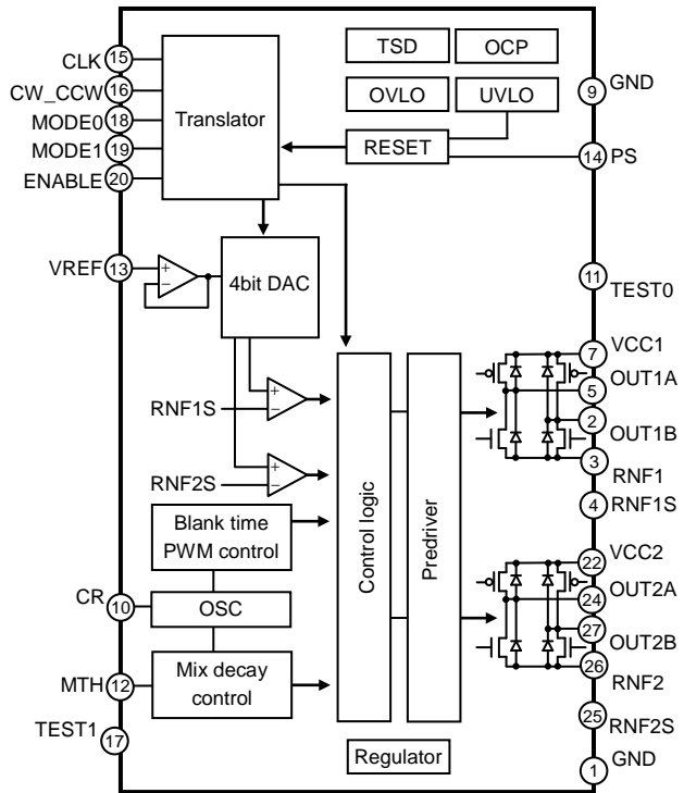
Figure.3 BD63511EFV ブロック図
