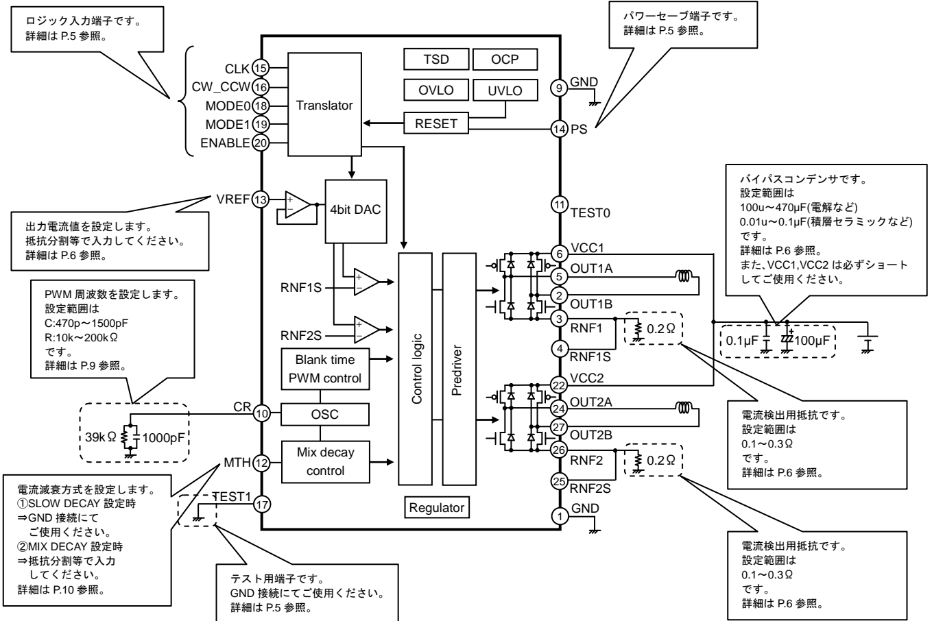
Figure.8 BD63511EFV ブロック図・応用回路図
