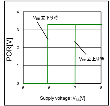
Figure 17. POR スレッシュロルド電圧 (Ta = 25 °C)
