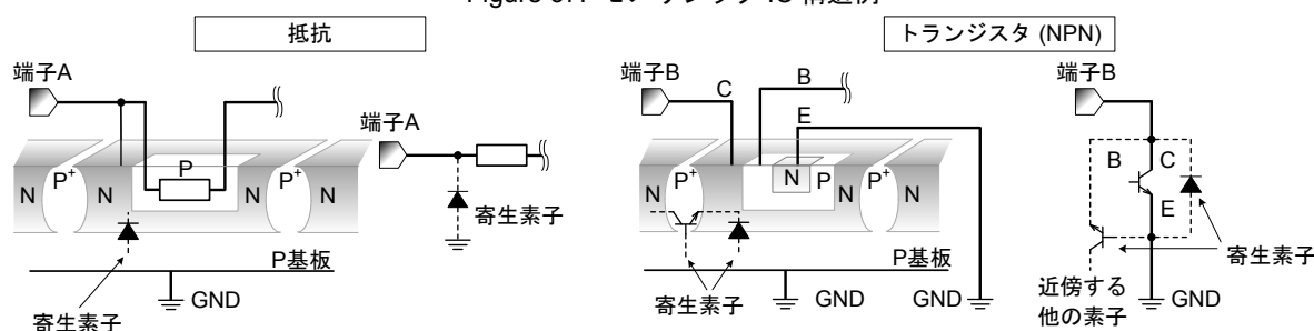
Figure 67. モノリシック IC 構造例
