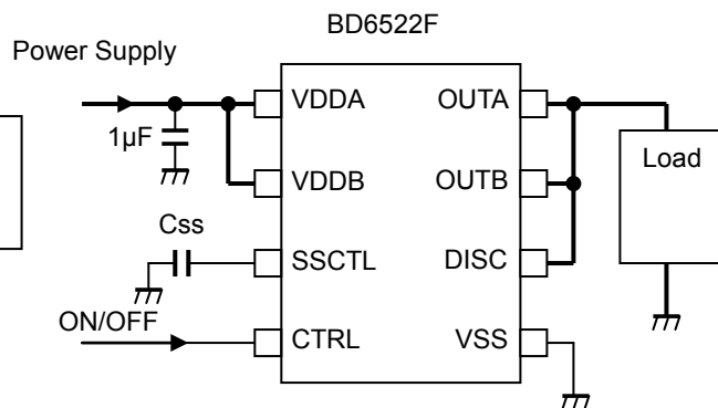
Figure 61. 電源スイッチ回路(BD6522F)
