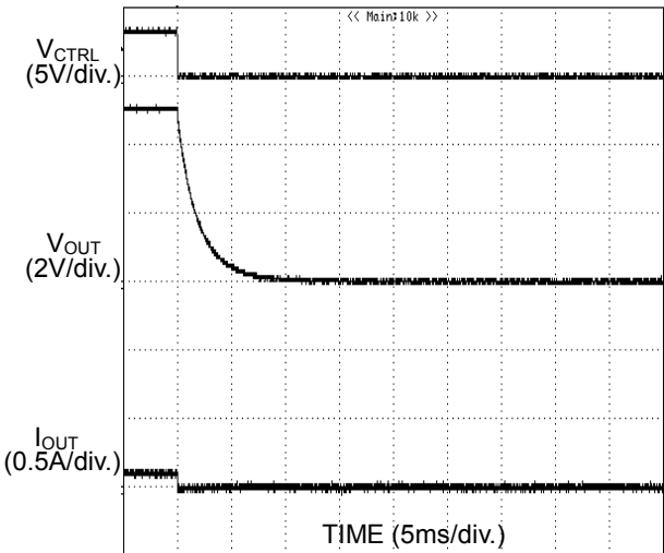
Figure 51. 立ち下り波形 (BD6520F)
