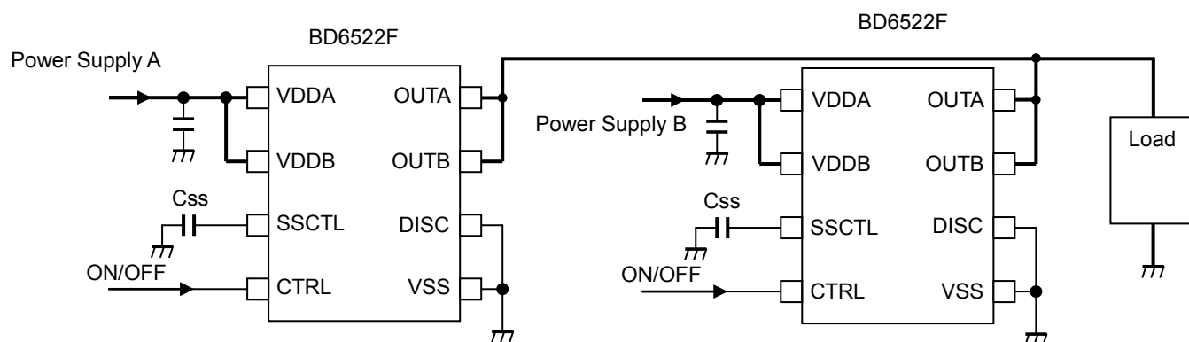
Figure 62. 2 電源の切り換えスイッチ回路(BD6522F)
