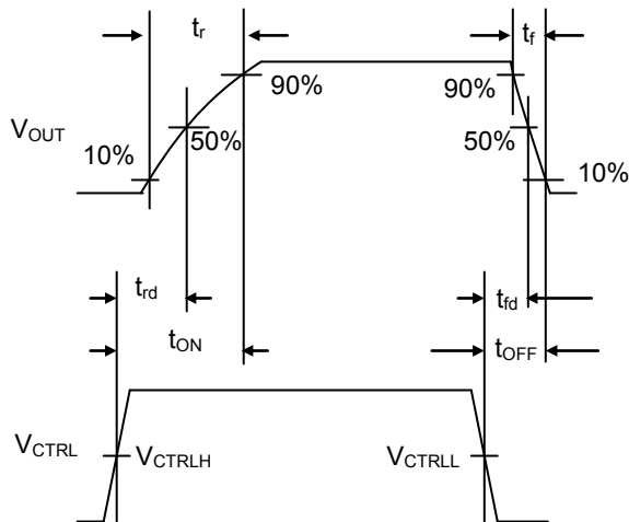
Figure 4. タイミングダイアグラム
