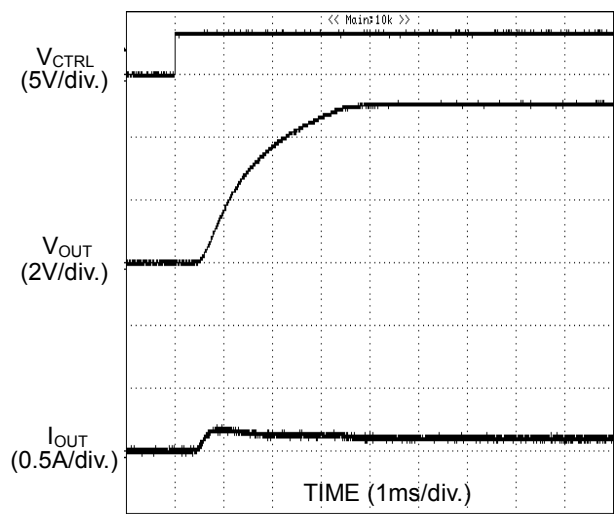
Figure 50. 立ち上り波形 (BD6520F)
