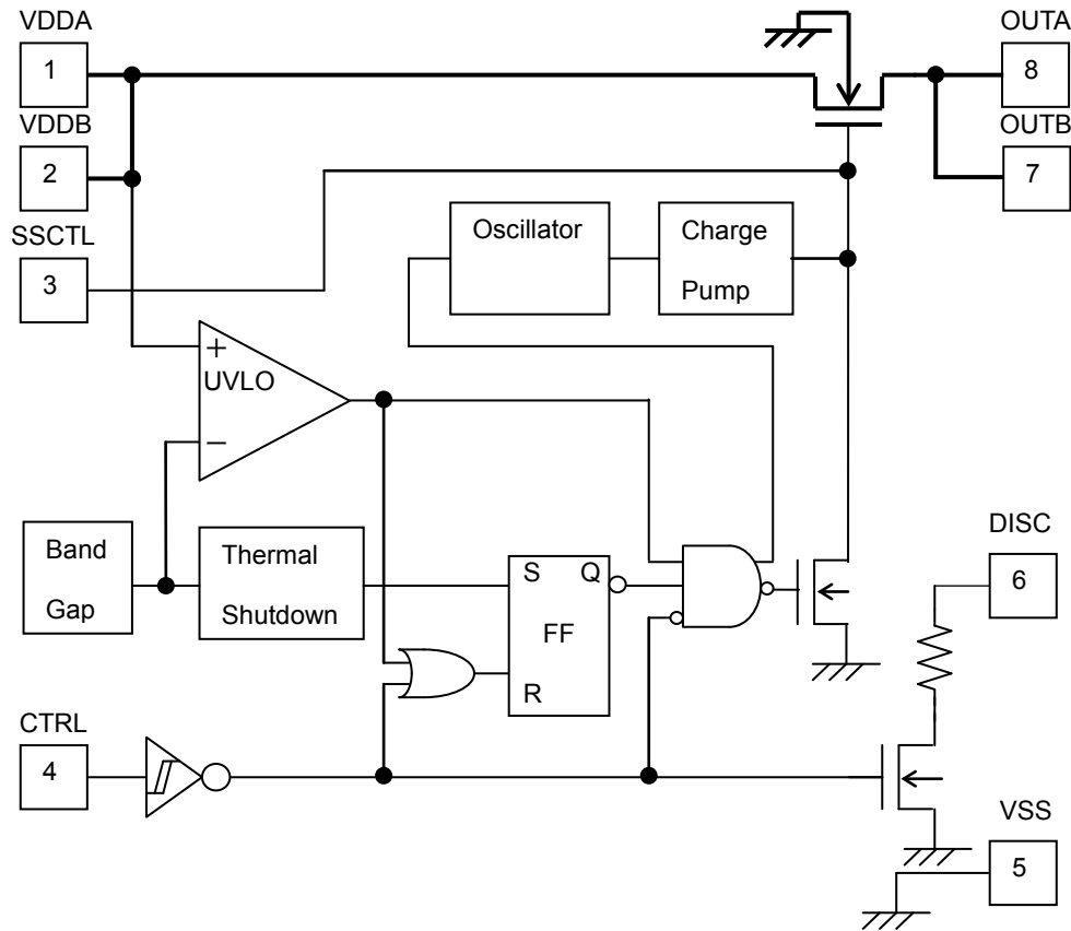
Figure 2. ブロック図 (BD6522F)
