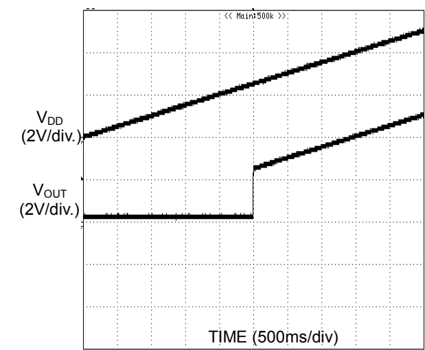
Figure 58. UVLO 動作( V_{DD} 上昇時)
