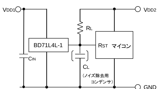
Figure 16. オープンドレイン出力タイプ
