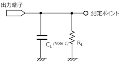
測定回路図 ( t_{PLH} , t_{PHL} )
