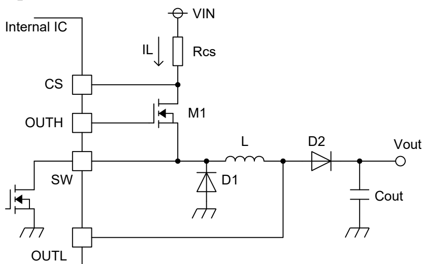
出力アプリケーション回路図（昇降圧構成の場合）
