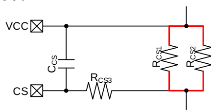
Figure 17. R_{CS} を並列に配置する場合
