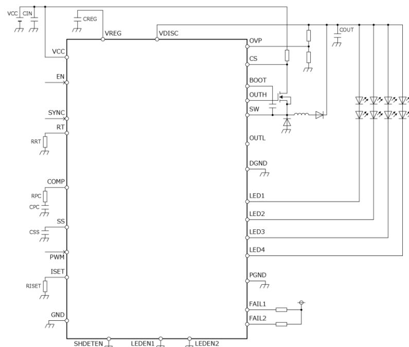
Figure 15. 降圧アプリケーション回路図
