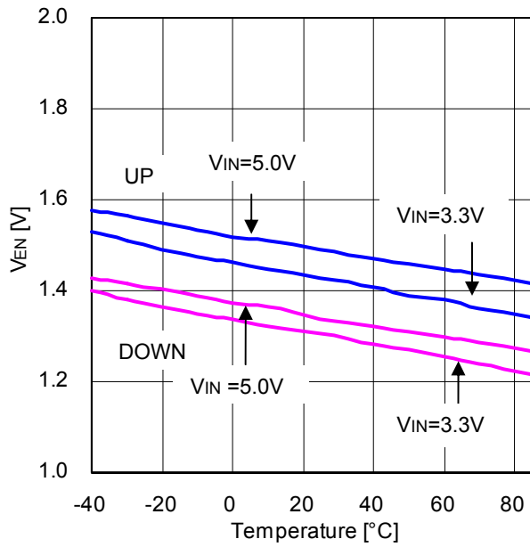
Figure 12. EN スレッシュホルド電圧 vs 温度
