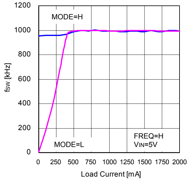
Figure 25. スイッチング周波数 vs 負荷電流
