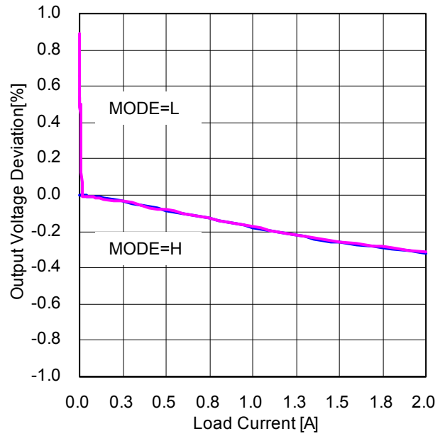
Figure 37. ロードレギュレーション ( V_{IN}=5V , V_{OUT}=1.2V , L=1.5\mu H , FREQ=H )
