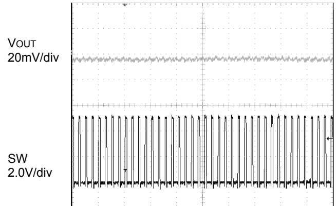
Figure 42. PWM 制御時 SW 波形) ( V_{IN}=5.0V , V_{OUT}=1.2V , I_{out}=2A )
