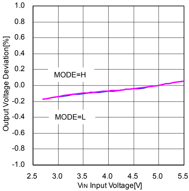
Figure 36. ラインレギュレーション ( V_{OUT}=1.2V , L=1.5\mu H , FREQ=H , I_{OUT}=2A )
