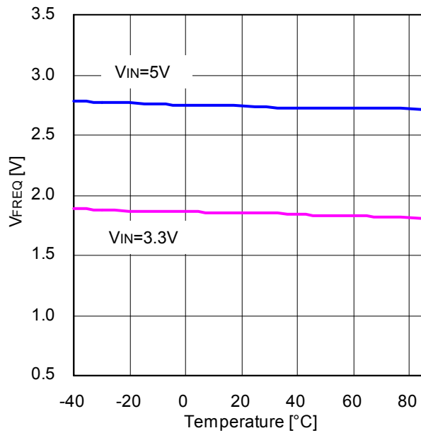
Figure 14. FREQ スレッシュホルド電圧 vs 温度
