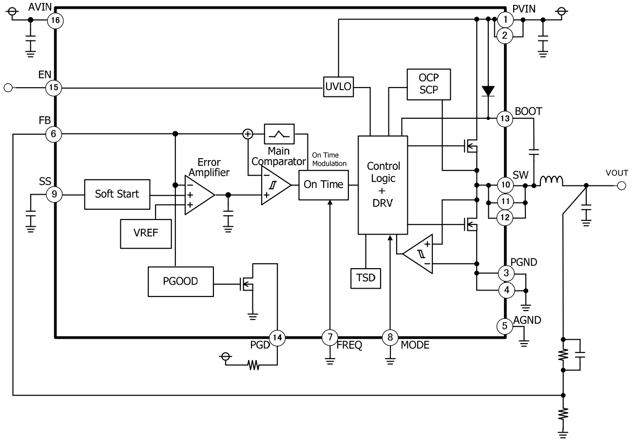
Figure 3. ブロック図
