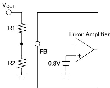
Figure 51. フィードバック抵抗回路
