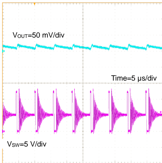
Figure 28. V_{OUT} リップル波形 ( V_{IN}=12\text{ V} , V_{OUT}=5\text{ V} , I_{OUT}=20\text{ mA} , C_{OUT}=10\text{ }\mu\text{F}\times 3 )
