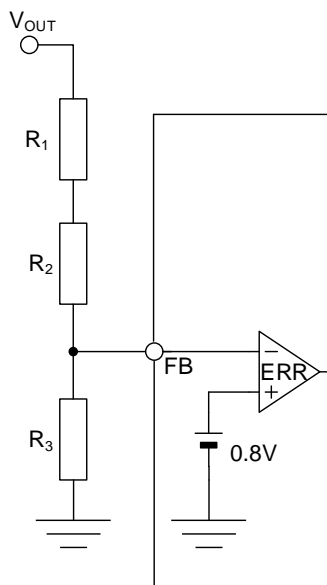
Figure 47. フィードバック抵抗回路
