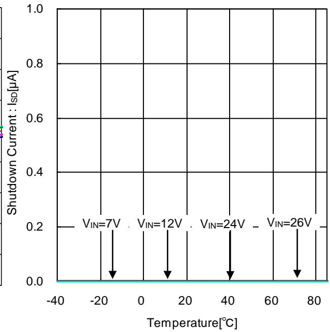
Figure 5. シャットダウン時回路電流 vs 周囲温度
