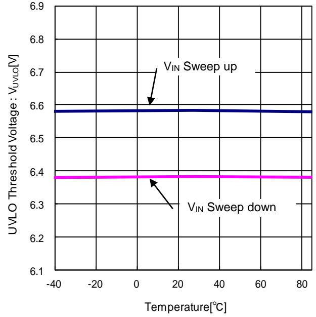
Figure 13. UVLO スレッシュヨルド電圧 vs 周囲温度
