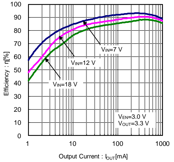
Figure 19. 効率 vs 出力負荷電流 ( V_{OUT}=3.3\text{ V} )
