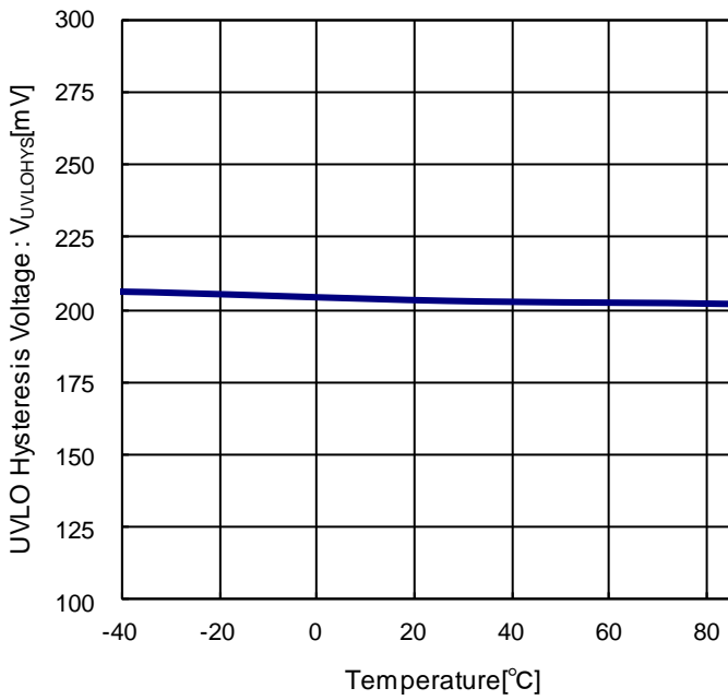
Figure 14. UVLO ヒステリシス電圧 vs 周囲温度
