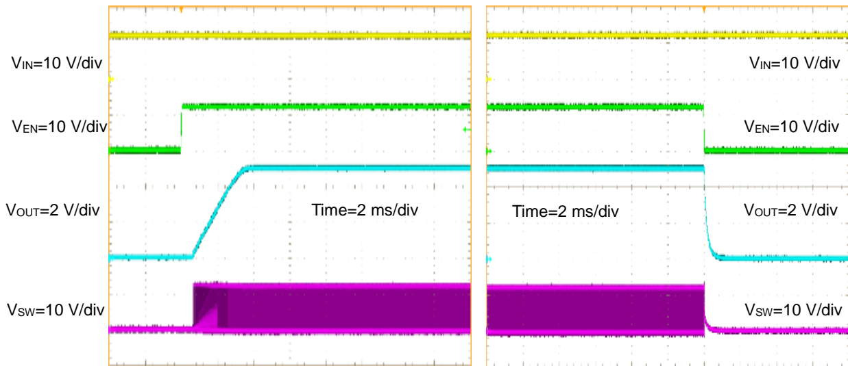
Figure 24. 起動波形 ( V_{EN}=0\text{ V}\rightarrow 5\text{ V} ) I_{OUT}=1.0\text{ A}
