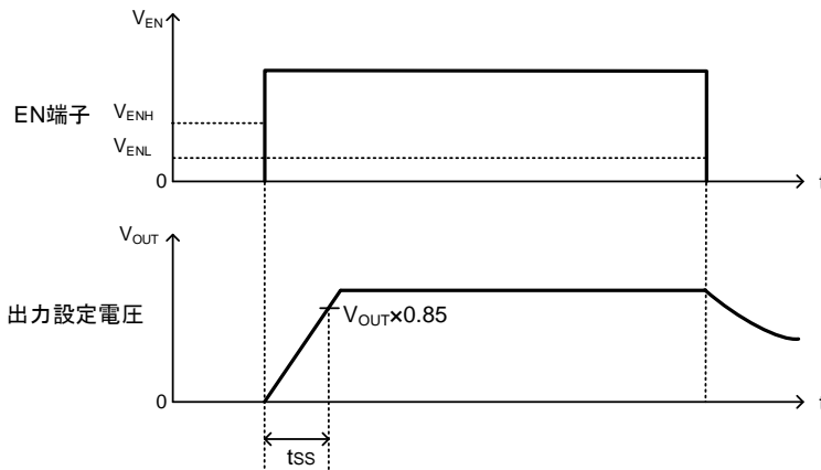
Figure 41. イネーブル制御タイミングチャート
