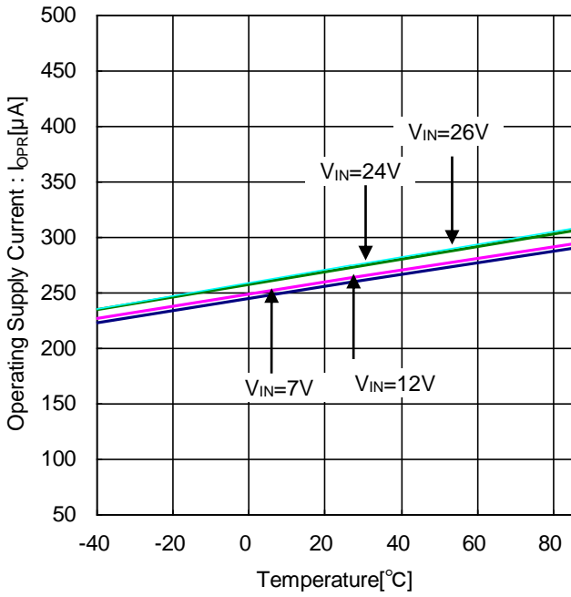
Figure 4. 静止時動作電流 vs 周囲温度
