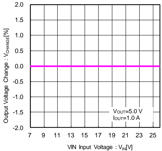
Figure 21. V_{OUT} ラインレギュレーション
