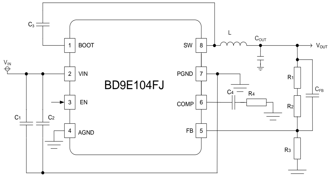
Figure 44. アプリケーション回路
