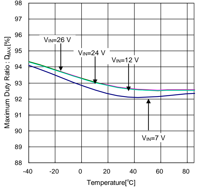
Figure 9. 最大デューティ比 vs 周囲温度
