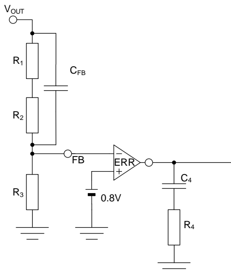
Figure 48. 位相補償回路
