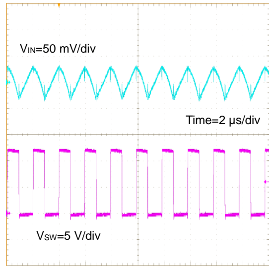
Figure 31. V_{IN} リップル波形 ( V_{IN}=12 \text{ V} , V_{OUT}=5 \text{ V} , I_{OUT}=1 \text{ A} )
