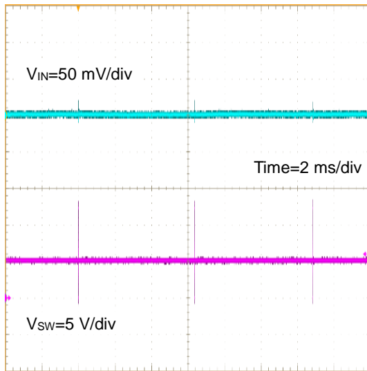
Figure 30. V_{IN} リップル波形 ( V_{IN}=12 \text{ V} , V_{OUT}=5 \text{ V} , I_{OUT}=0 \text{ A} )
