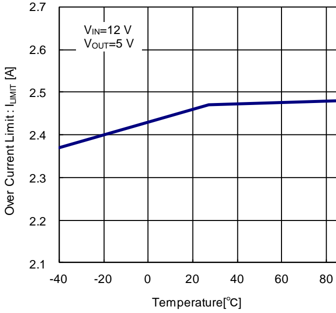
Figure 12. 電流制限スレッシュヨルド vs 周囲温度
