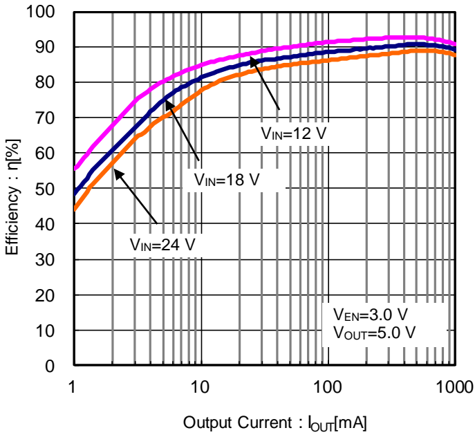
Figure 18. 効率 vs 出力負荷電流 ( V_{OUT}=5.0\text{ V} )
