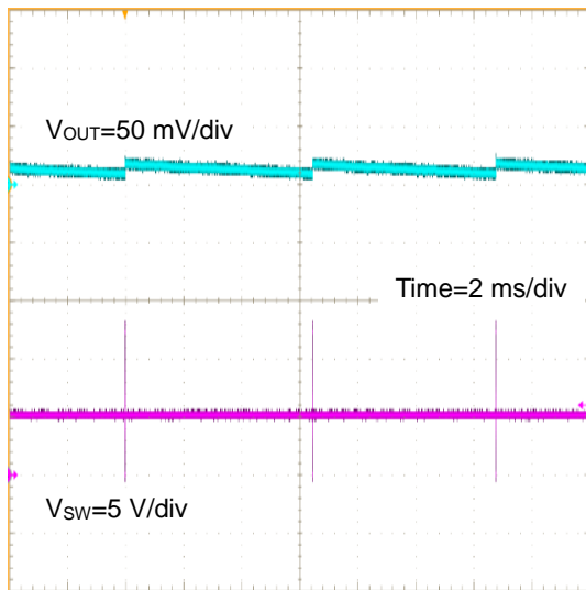
Figure 26. V_{OUT} リップル波形 ( V_{IN}=12\text{ V} , V_{OUT}=5\text{ V} , I_{OUT}=0\text{ A} , C_{OUT}=10\text{ }\mu\text{F}\times 3 )
