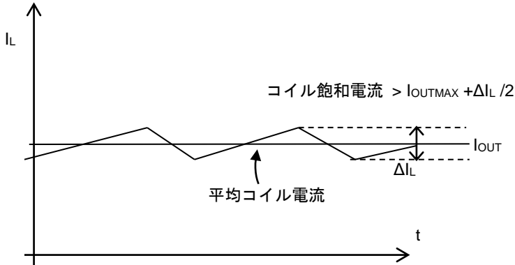
Figure 45. インダクタに流れる電流波形
