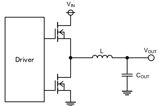
Figure 46. 出力 LC フィルタ回路
