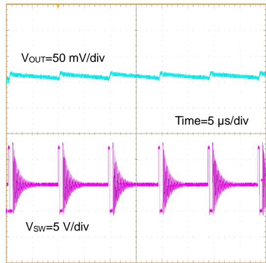
Figure 27. V_{OUT} リップル波形 ( V_{IN}=12\text{ V} , V_{OUT}=5\text{ V} , I_{OUT}=10\text{ mA} , C_{OUT}=10\text{ }\mu\text{F}\times 3 )
