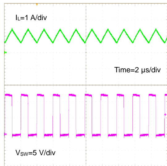
Figure 33. SW 波形 ( V_{IN}=12 \text{ V} , V_{OUT}=5 \text{ V} , I_{OUT}=1 \text{ A} )
