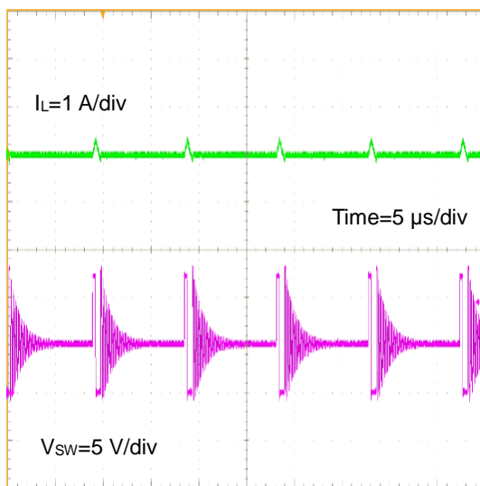
Figure 32. SW 波形 ( V_{IN}=12 \text{ V} , V_{OUT}=5 \text{ V} , I_{OUT}=10 \text{ mA} )
