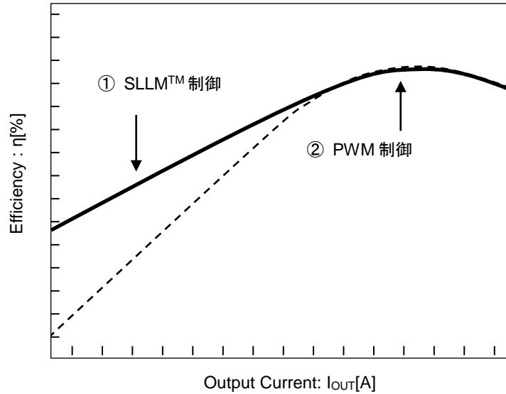
Figure 38. 効率特性 (SLLM™ 制御、PWM 制御)
