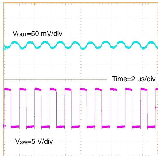
Figure 29. V_{OUT} リップル波形 ( V_{IN}=12\text{ V} , V_{OUT}=5\text{ V} , I_{OUT}=1\text{ A} , C_{OUT}=10\text{ }\mu\text{F}\times 3 )
