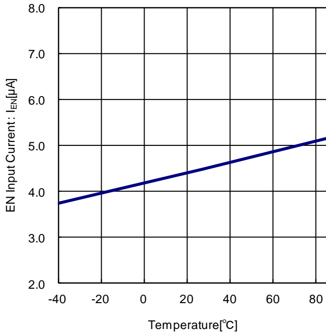
Figure 16. EN 流入電流 vs 周囲温度
