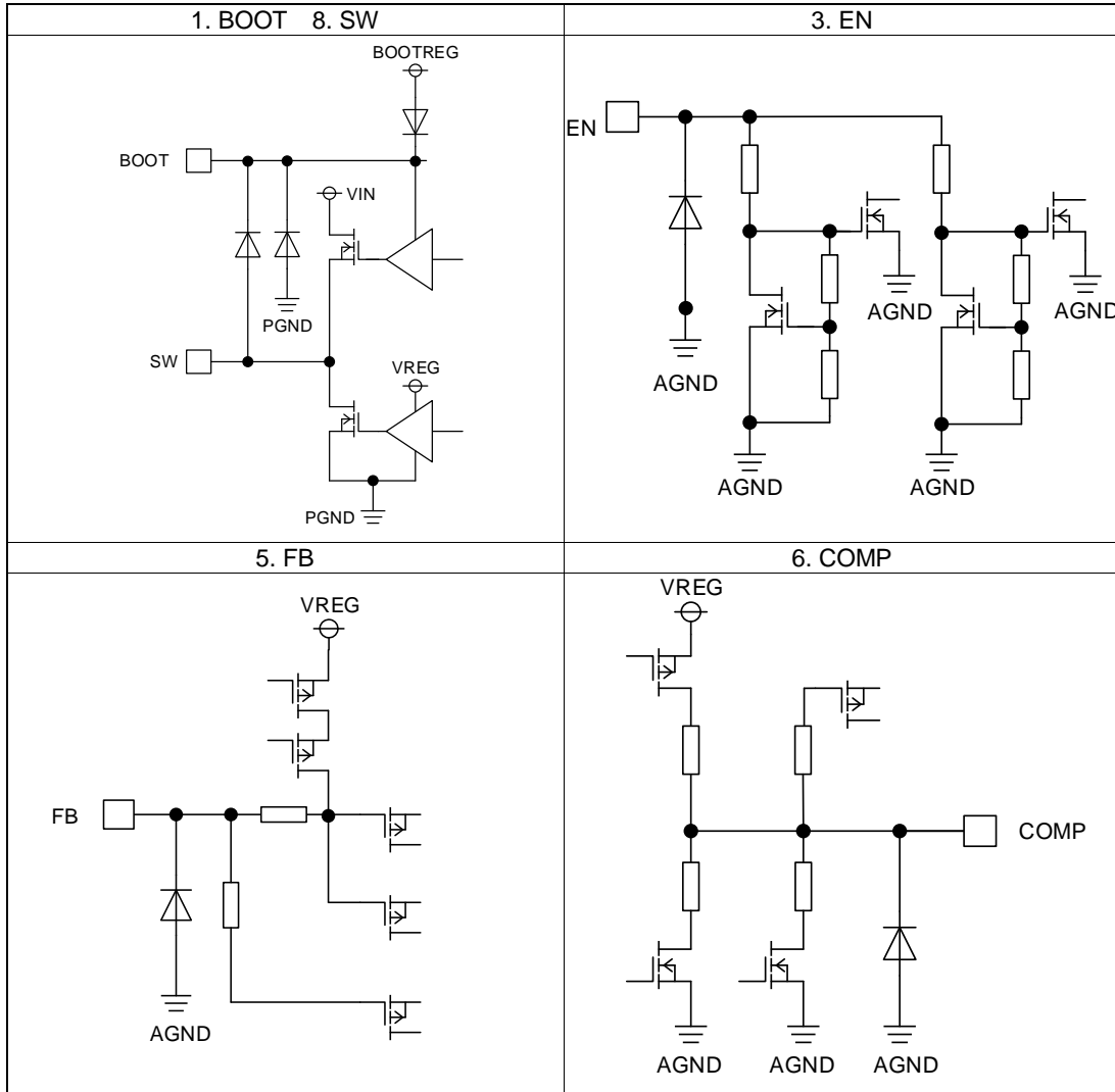
Figure 52. 入出力等価回路図
