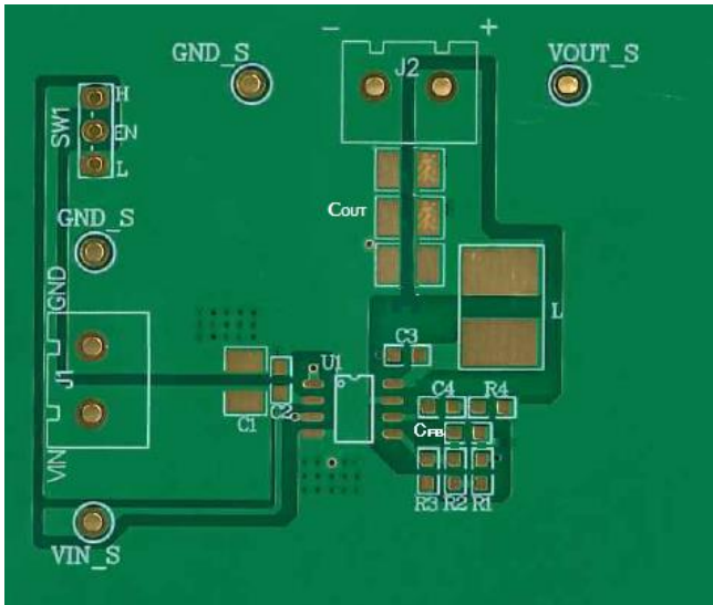
Top Layer
