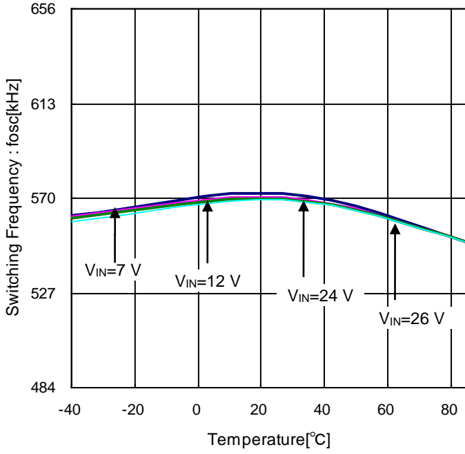
Figure 8. スイッチング周波数 vs 周囲温度
