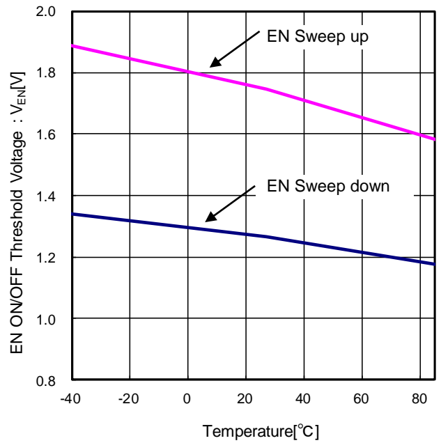
Figure 15. EN ON/OFF スレッシュヨルド電圧 vs 周囲温度
