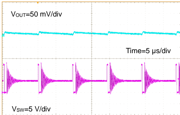
Figure 39. SLLM™ 制御時 SW 波形 (V IN =12 V, V OUT =5.0 V, I OUT =10 mA)
