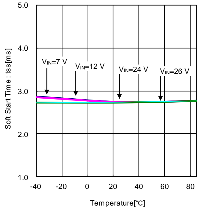
Figure 17. ソフトスタート時間 vs 周囲温度
