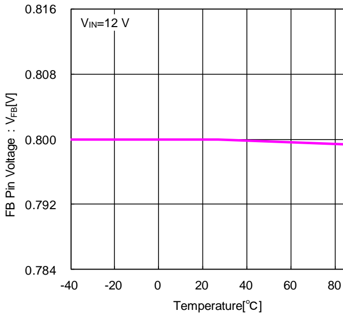
Figure 6. FB 端子電圧 vs 周囲温度
