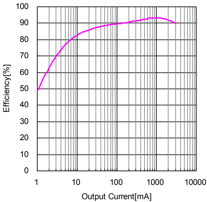
Figure 48. 効率 vs 出力負荷電流 ( V_{IN}=12V , V_{OUT} = 5.0V , R_3=15k\Omega , C_1=18pF )
