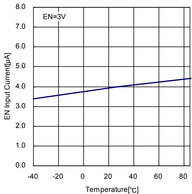
Figure 15. EN 端子流入電流 vs 周囲温度
