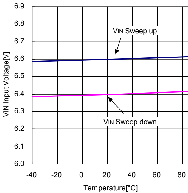
Figure 12. UVLO スレッシュヨルド vs 周囲温度
