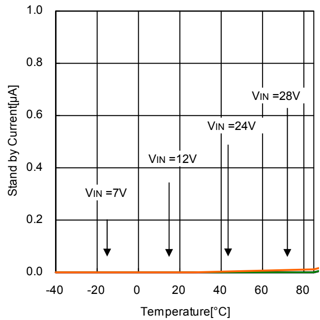
Figure 5. スタンバイ電流 vs 周囲温度
