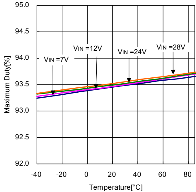
Figure 9. 最大デューティ比 vs 周囲温度
