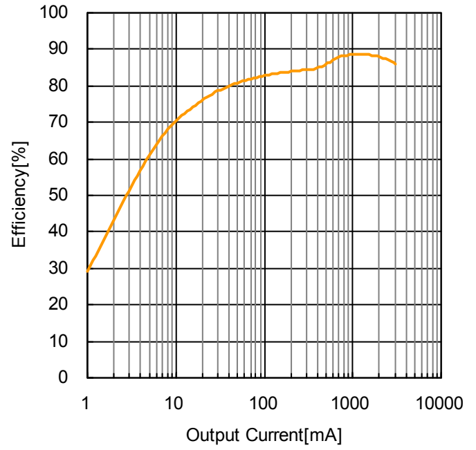
Figure 40. 効率 vs 出力負荷電流 ( V_{IN}=24V , V_{OUT} = 5.0V , R_3=10k\Omega )
