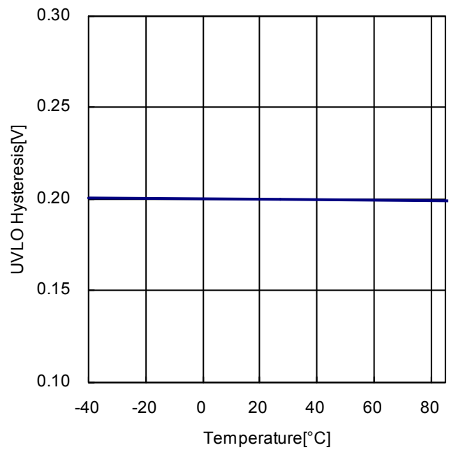
Figure 13. UVLO ヒステリシス vs 周囲温度
