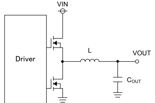
Figure 76. 出力 LC フィルタ回路
