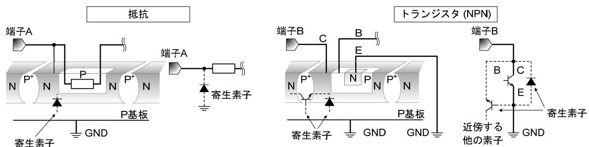
Figure 81. モノリシック IC 構造例
