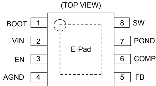
Figure 2. 端子配置図
