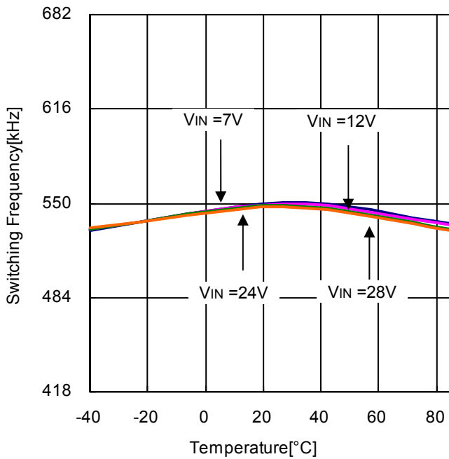
Figure 8. スイッチング周波数 vs 周囲温度
