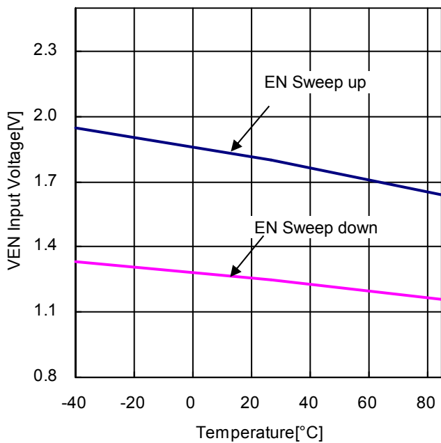
Figure 14. EN ON/OFF スレッシュヨルド vs 周囲温度
