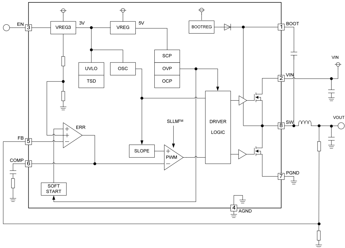
Figure 3. ブロック図
