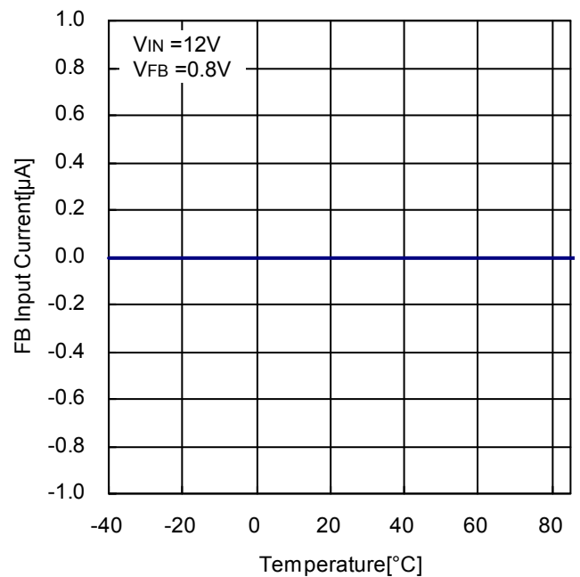
Figure 7. FB 入力バイアス電流 vs 周囲温度
