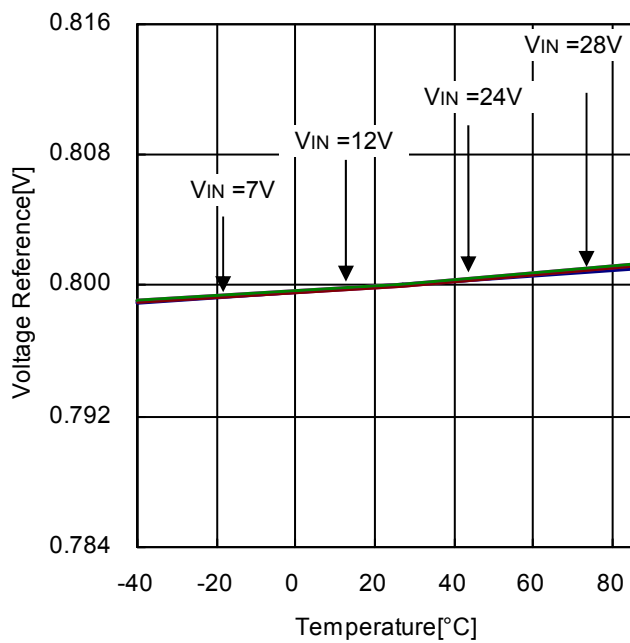
Figure 6. 基準電圧 vs 周囲温度
