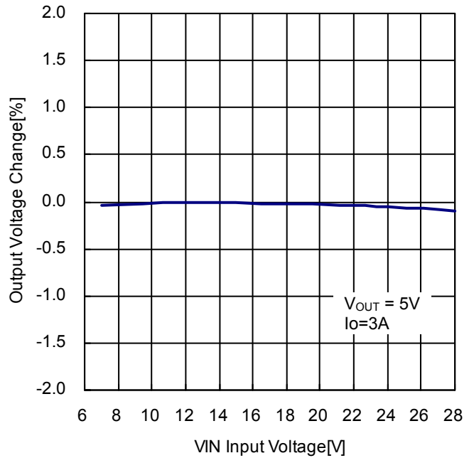
Figure 29. VOUT ラインレギュレーション Vout = 5V
