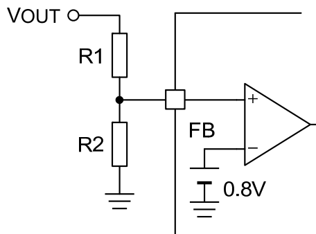
Figure74. フィードバック抵抗回路
