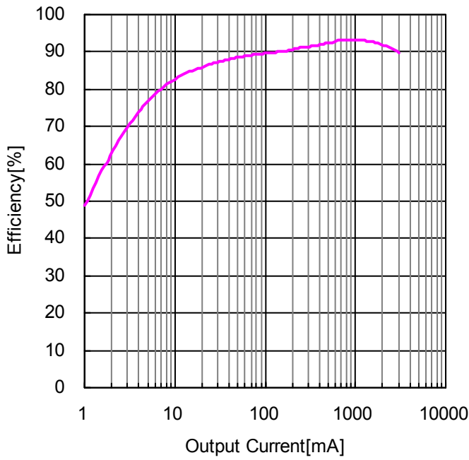
Figure 39. 効率 vs 出力負荷電流 ( V_{IN}=12V , V_{OUT} = 5.0V , R_3=10k\Omega )
