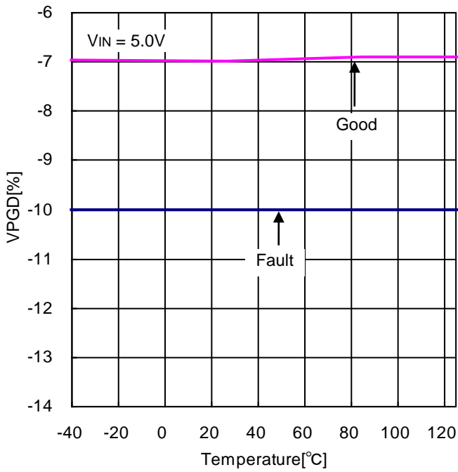
Figure 16. PGD 電圧 vs 温度
