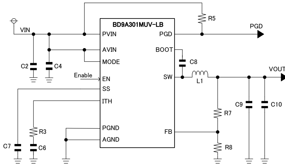
Figure 48. アプリケーション回路
