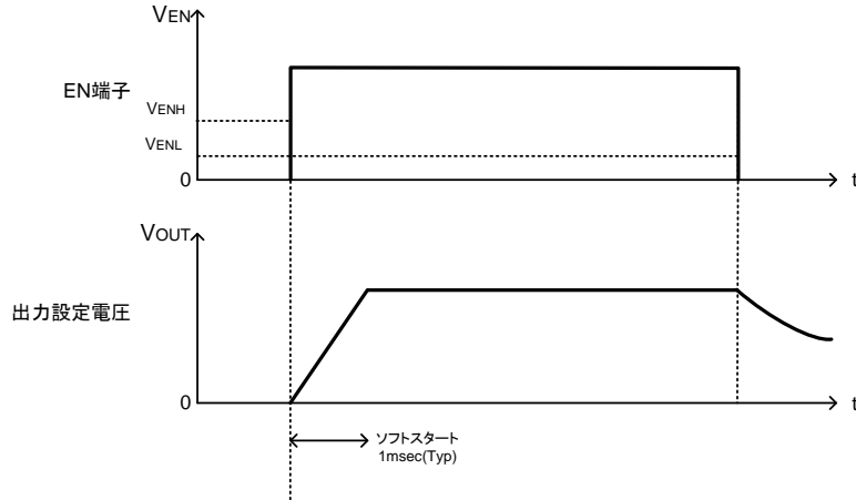
Figure 44. イネーブル制御中の ON/OFF 切り替え
