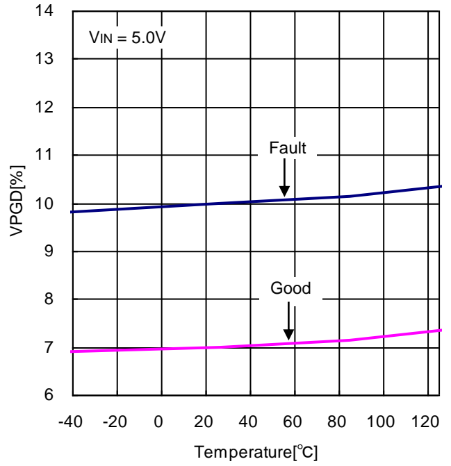
Figure 17. PGD 電圧 vs 温度
