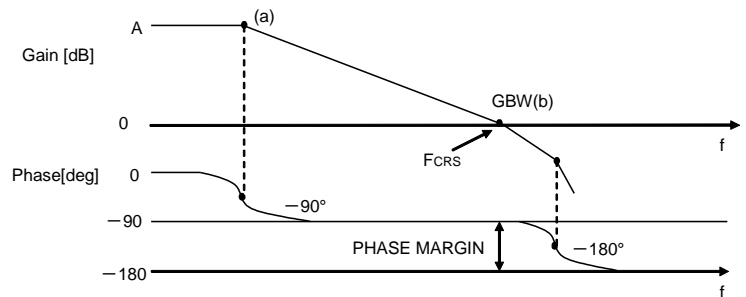
Figure 53. ボード線図
