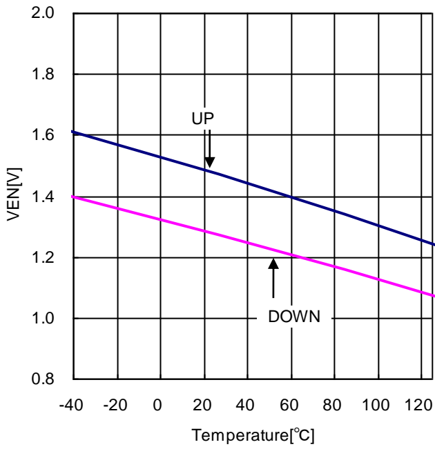
Figure 20. EN スレッシュヨルド電圧 vs 温度
