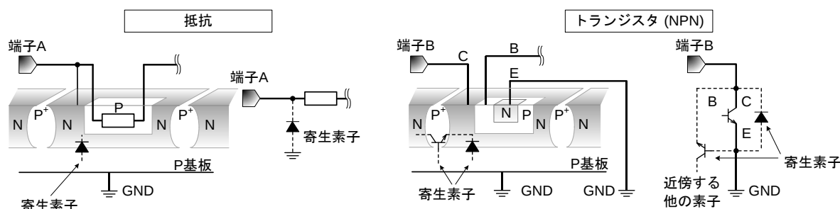
Figure. モノリシック IC 構造例
