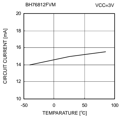
Fig. 18 回路電流—周囲温度
