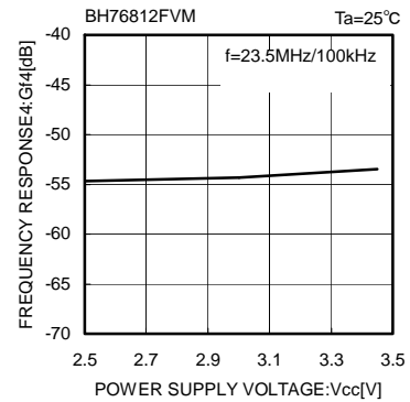
Fig. 29 周波数特性 4—電源電圧
