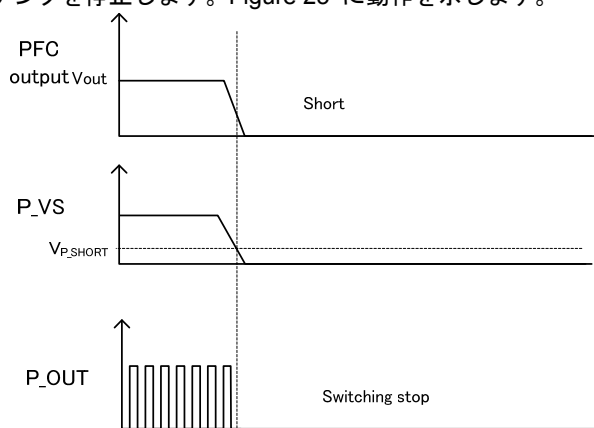
Figure 25. P_VS ショート保護動作
