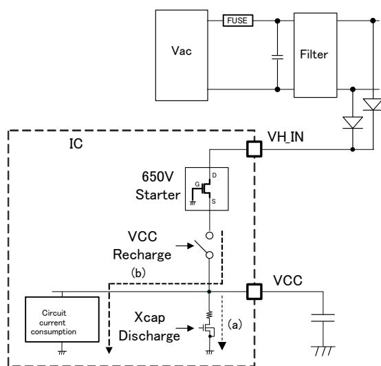
Figure 4. 起動回路ブロック図
