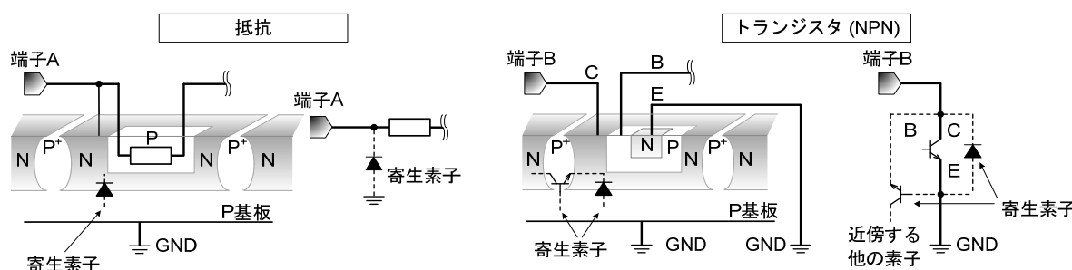
Figure 42. モノリシック IC 構造例
