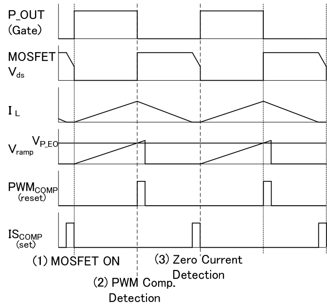
Figure 22. スイッチング動作タイミングチャート
