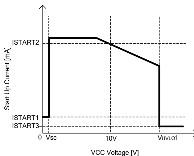
Figure 5. 起動電流 vs VCC 電圧
