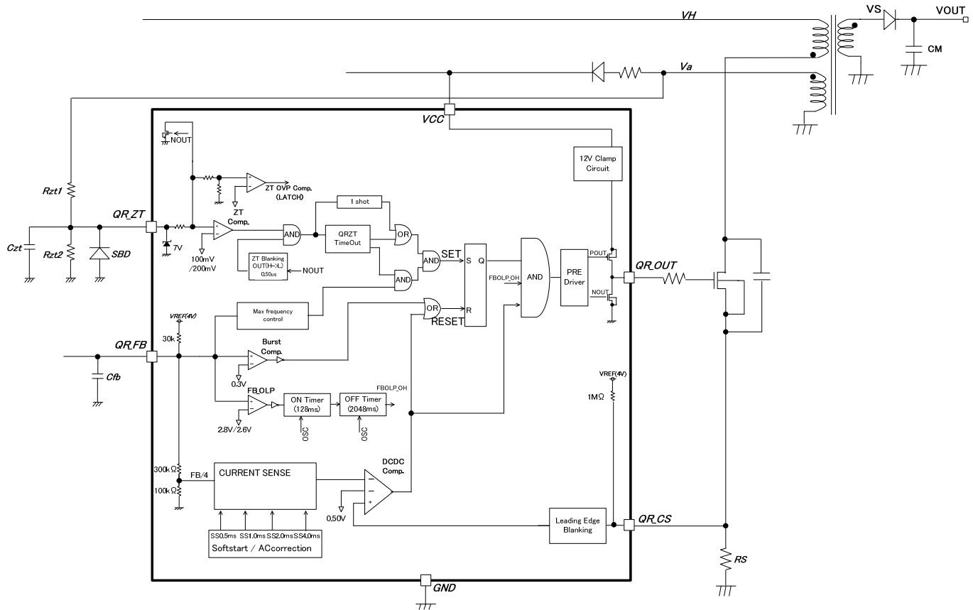
Figure 13. DC/DC 動作ブロック図
