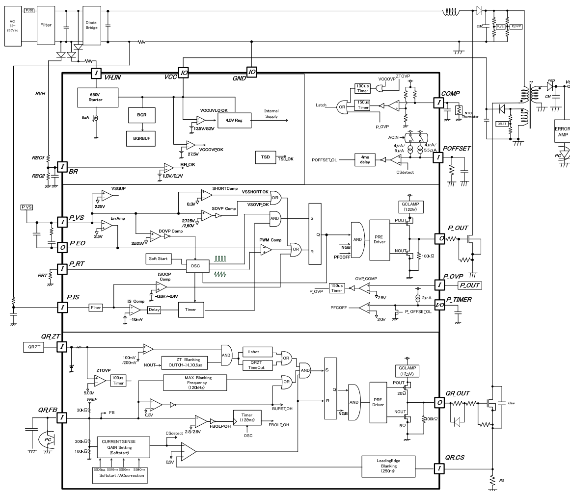
Figure 3.ブロック図
