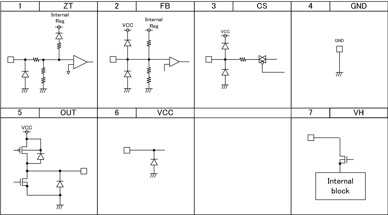
Figure-3 入出力等価回路図
