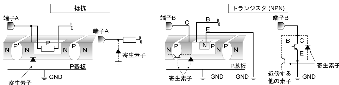
Figure-28. モノリシック IC 構造例
