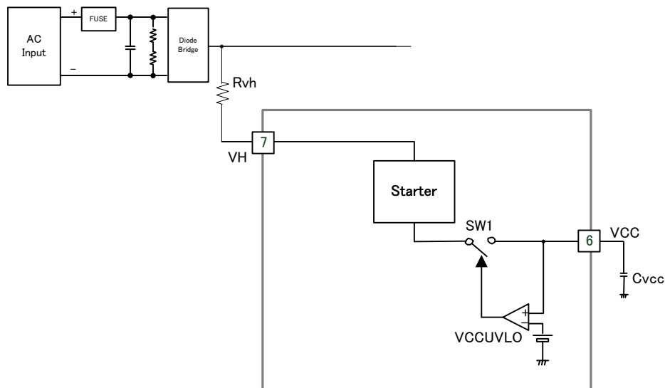
Figure-5. 起動回路ブロック図
