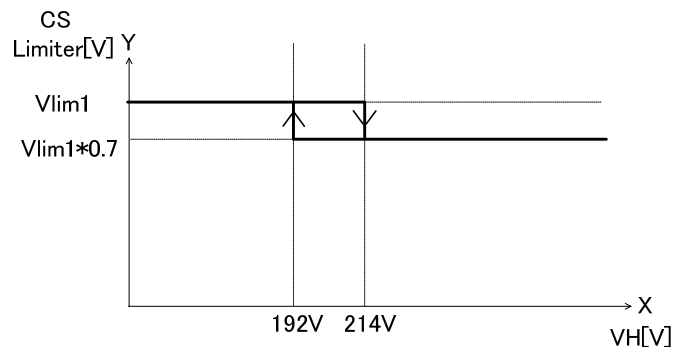
Figure-21 CS 切り換え例 V_H 電圧 - CS 電圧特性
