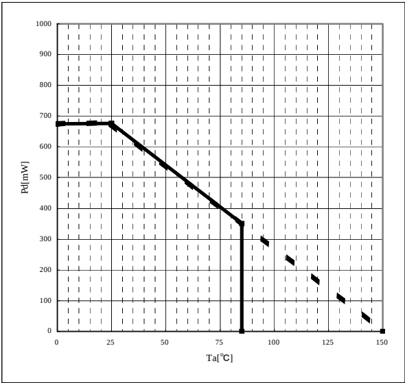
Figure-27 SOP-J7S 熱軽減特性
