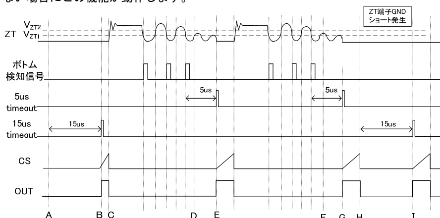
Figure-23 ZTタイムアウト機能
