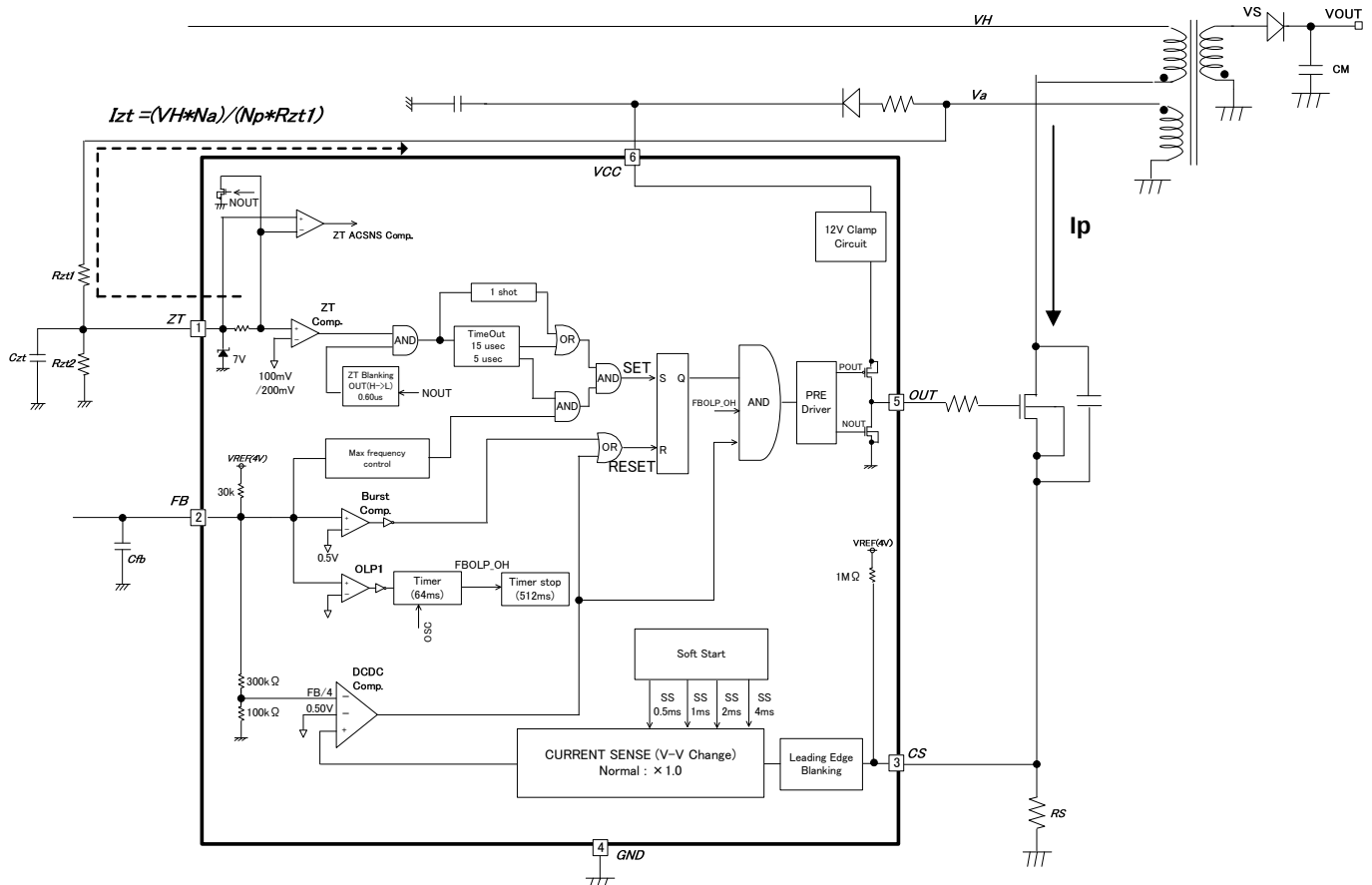
Figure-14 IC 内部 QR 動作ブロック図
