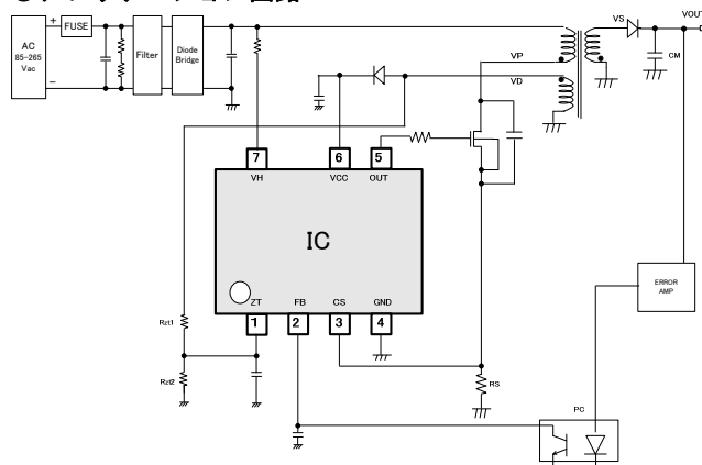
Figure-1. アプリケーション回路
