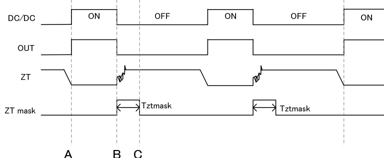
Figure-22 ZTトリガマスク機能
