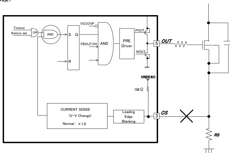
Figure-24 CS オープン保護回路
