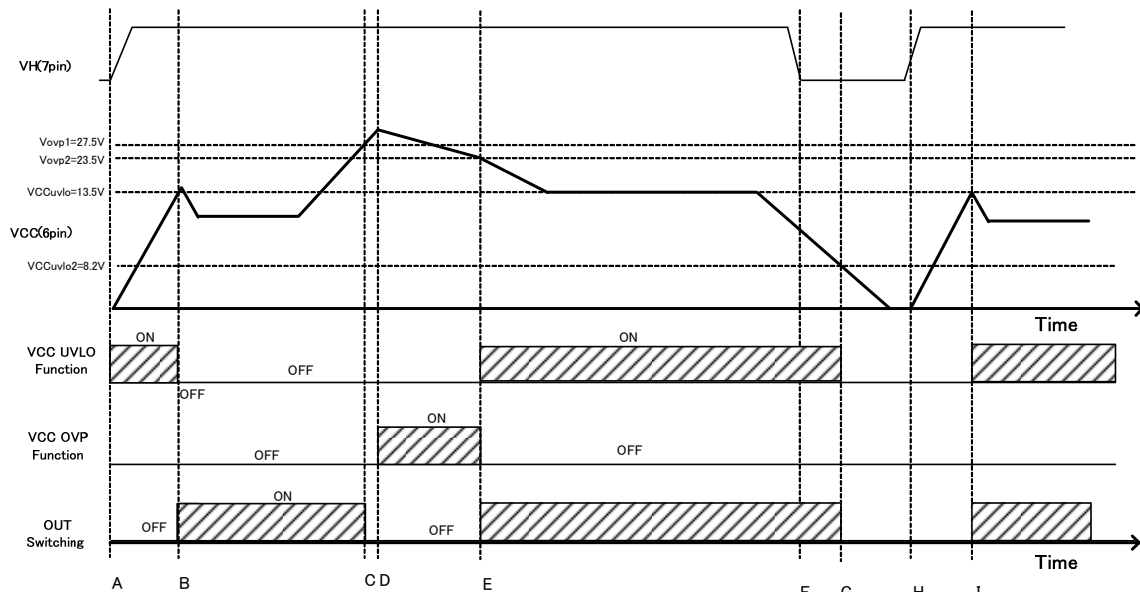
Figure-11 VCC UVLO / OVP タイムチャート
