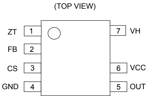
Figure-2 SOP-J7 パッケージ外形図
