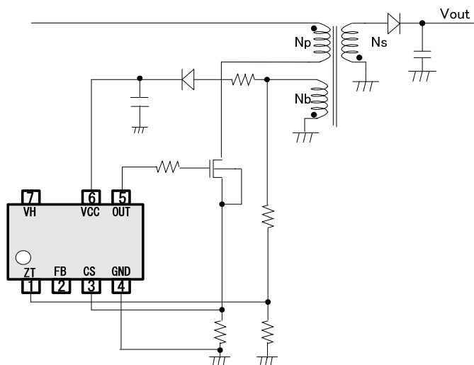
Figure-12 VCCOVP 設定方法
