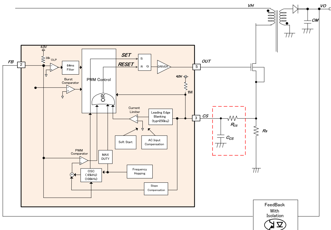
Figure-17. CS 端子周辺回路
