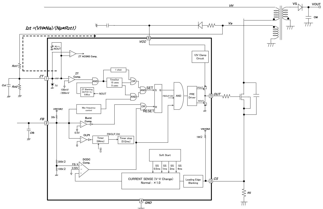
Figure-18 CS 切り換え電流ブロック図
