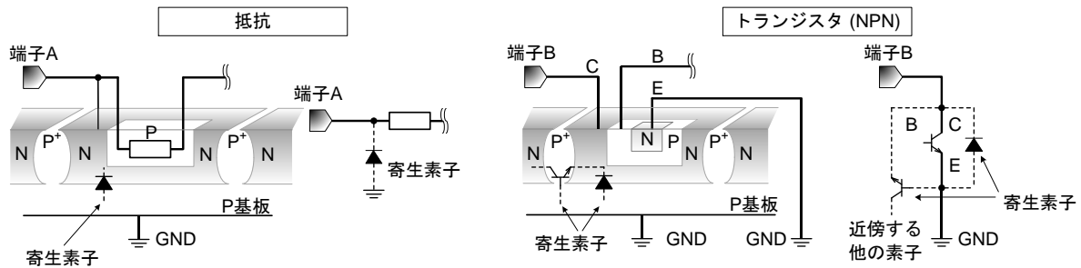
Figure 38. IC 構造例
