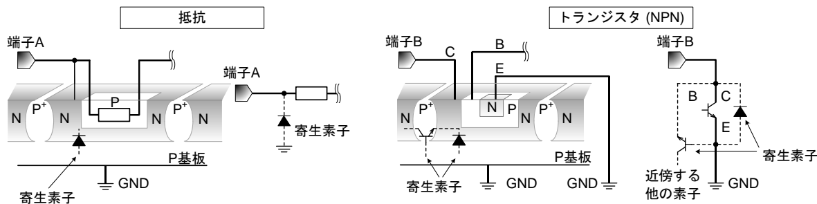
Figure 33. IC 構造例
