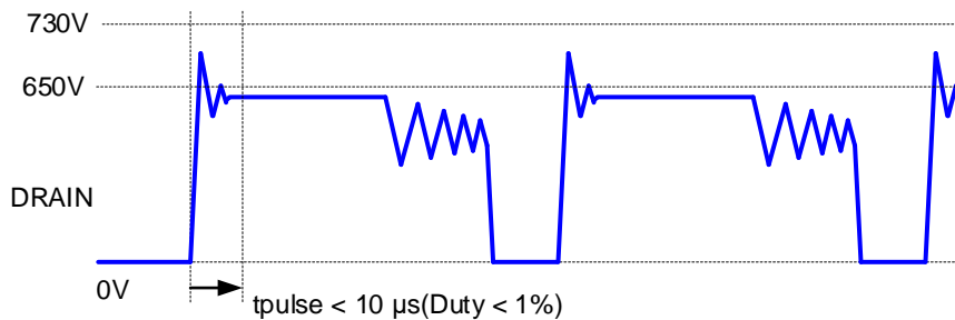
Figure 34. ドレイン端子リングング波形
