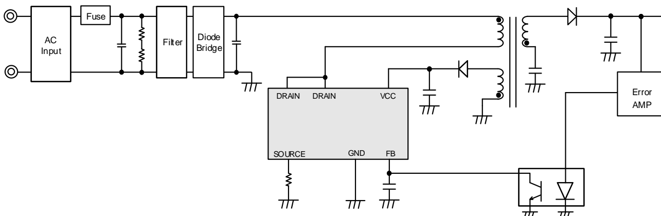
Figure 33. フライバックアプリケーション図
